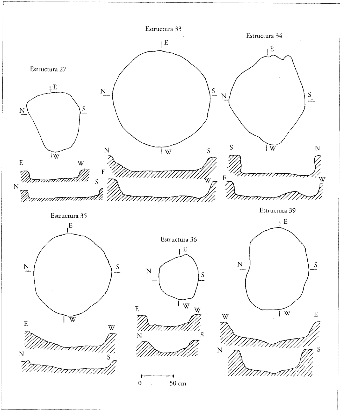
FIGURA 4. Representació, en planta i seccions, d'algunes de les fosses documentades durant l'excavació de la necròpolis del Pla de la Bruguera.
