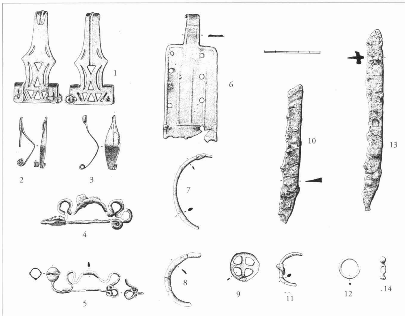
FIGURA 6. Objectes metàl·lics documentats a la necròpolis del Pla de la Bruguera: 1) sivella de placa romboïdal feta de bronze i amb anelles de ferro; 2-3) fibules del tipus «golf de Lleó», fetes de bronze i ferro; 4-5) fibules d'arc serpentiforme fetes de ferro; 6) sivella de placa rectangular feta de bronze i amb anelles de ferro; 7-8) braçalets fetes de bronze; 9) rodeta circular feta de bronze; 10) ganivet de ferro de tipus «Gran Bassin»; 11-12) anells/anelles fetes de bronze; 13) ganivet de ferro de tipus «Gran Bassin»; 14) cap d'agulla de pes feta de bronze (Dibuixos: J. Ariza).
