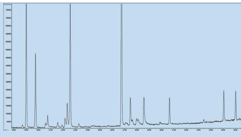
Figura 9. Exemple de la identificació dels composts presents al romani.
