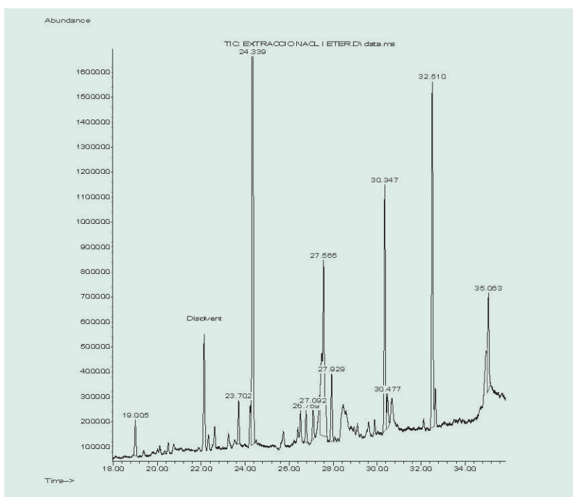
Figura 13. Cromatograma de l'extracte del licor.
