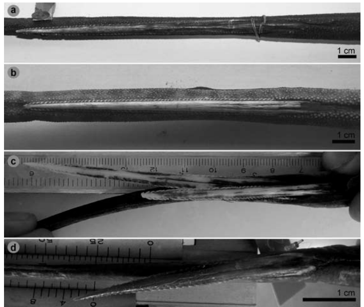
Figura 3: Detalls d'agullons caudals de rajades actuals: a, Dasyàtid indeterminat; b, Myliobatid Myliobatis narinaris ; c, doble agulló en Myliobatis aquila ; d, Dasyatis pastinaca . Les fotos de (a), (b), (d) van ser preses al Museu de Ciències Naturals de Barcelona i (c) a la Unitat de Zoologia de la Universitat Autònoma de Barcelona. (JOSEP MARMÍ)
