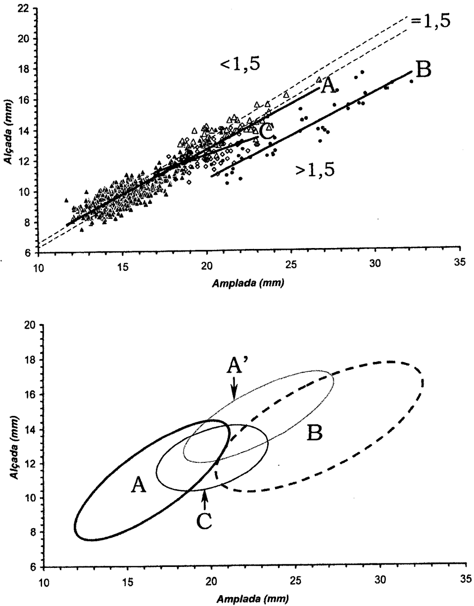
Fig. 5. Relació entre l'amplada i l'alçada de la closca d' I. pyrenaicus (la recta de regressió A Y = 0,5753X + 1,0989 ( R=0,9232 ) inclou els exemplars actuals i fòssils; el·lipse A i triangles negres: closques actuals; el·lipse A' i triangles blancs: closques fòssils), I. balearicus (cercles petits, recta de regressió i el·lipse B) i I. tanitianus (quadrats petits inclinats, recta de regressió i el·lipse C). Les línies discontinües representen la separació entre els tres rangs corresponents a la relació entre l'amplada i l'alçada.
