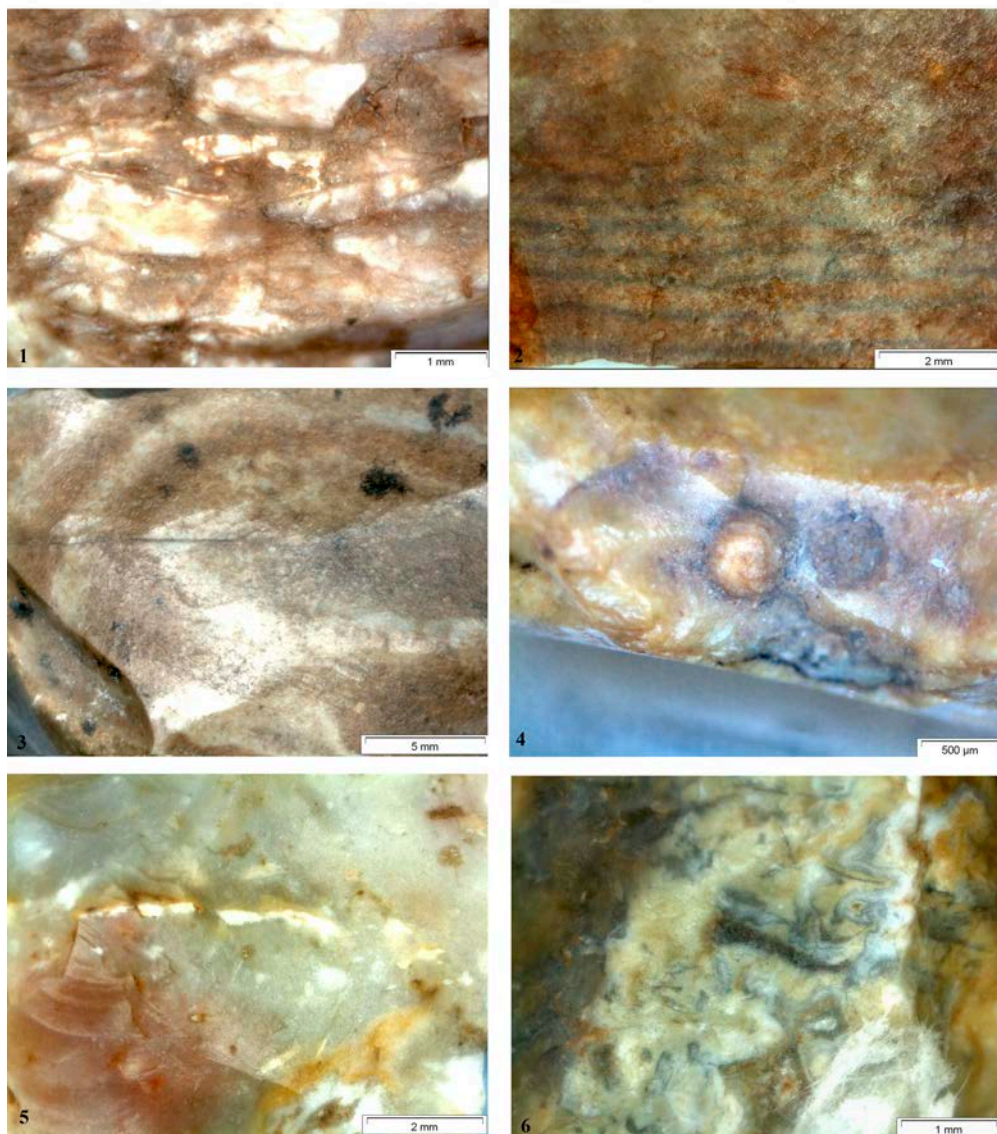
Fig. 3. Principales tipos de sílex determinado. 1) Sílex procedente de medios sedimentarios continentales/sílex evaporítico: lenticulas de yeso. 2) Sílex de medios sedimentarios de aguas de baja salinidad/lacustres-palustres: sílex de estructura bandeada. 3) Sílex con anillos de Liesegang, 4) Oogonio de carofito incluido en el sílex. 5) Sílex de tipo mudstone . 6) Sílex de crecimiento en filones/venas: sílex de tipo calcedónico.
