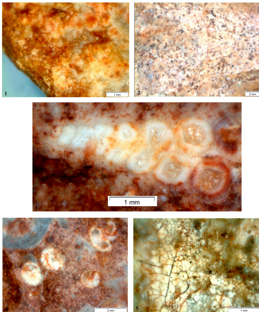
Fig. 4. Principales tipos de sílex determinado. 1) Sílex de crecimiento en filones/venas: sílex de tipo esferulítico. 2) Sílex de medio indeterminable: sílex de textura moteada. 3-4) Sílex con contenido micropaleontológico con gasterópodos en sección longitudinal y transversal, respectivamente. 5) Sílex termoalterado con craquelación.
