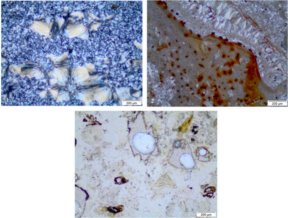
Fig. 5. Láminas delgadas de tres muestras de la Dolina de l'Esquerda de les Alzines. 1) LP 335: sílex continental/evaporítico, matriz de microcuarzo y esferulitas relleno de cavidades. 2) LP 400: raspador de sílex calcedónico, con bandas de matriz micrítica atravesadas por bandas calcedónicas. 3) LP 851: sílex moteado, matriz micrítica con Pattellina .
