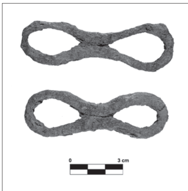
Lámina XV. Embocaduras de bocado, elementos de una cabezada parcialmente metálica (ver Lám. XIV y Fig. 13). Alcoi, 2630 y 2631.
