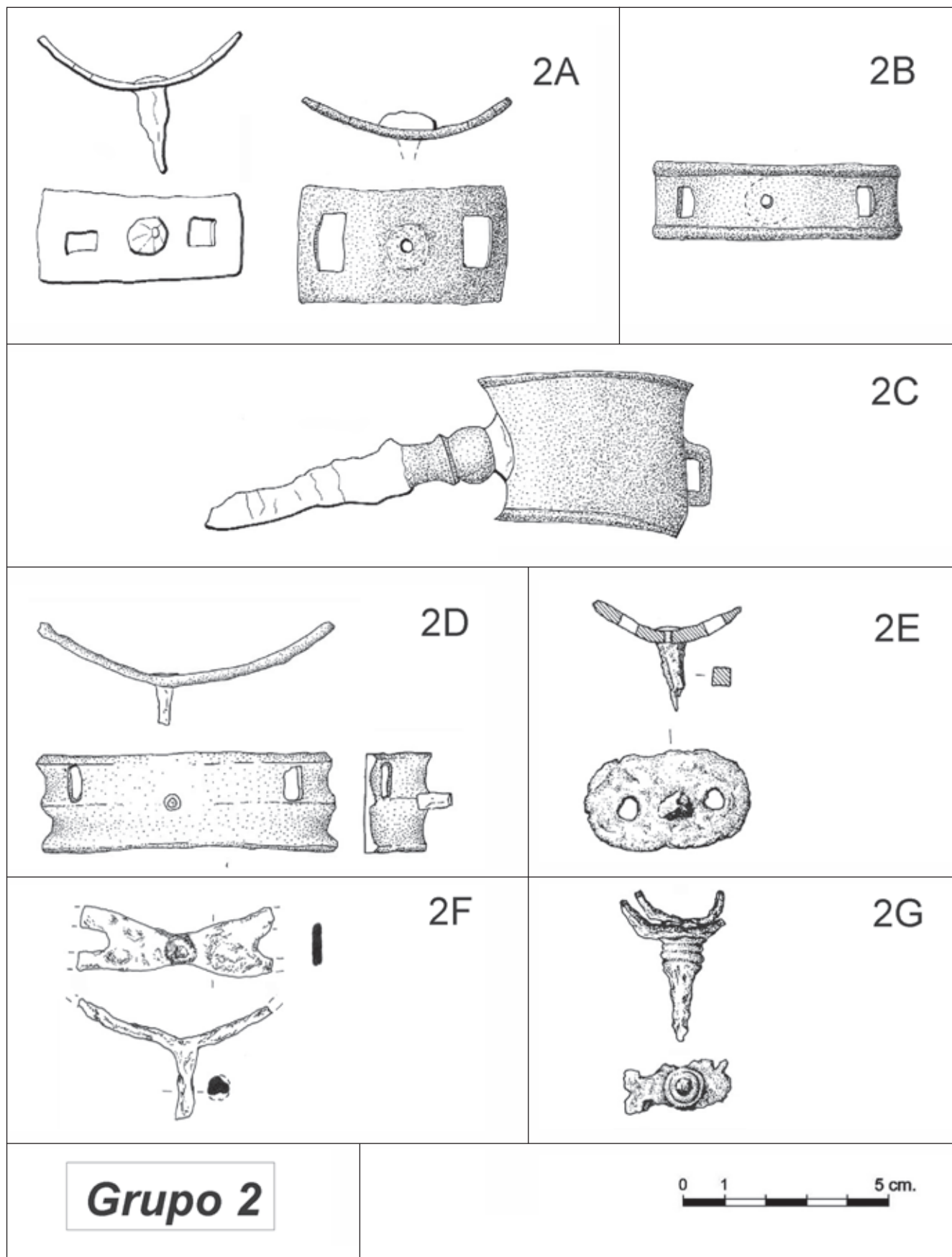
Figura 3. Tipos de espuela del Grupo 2 (espuelas rígidas de placa metálica).
