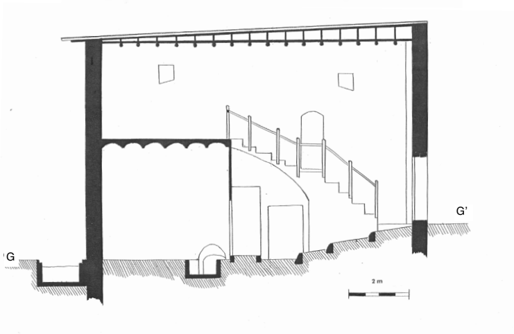
Secció G-G'
