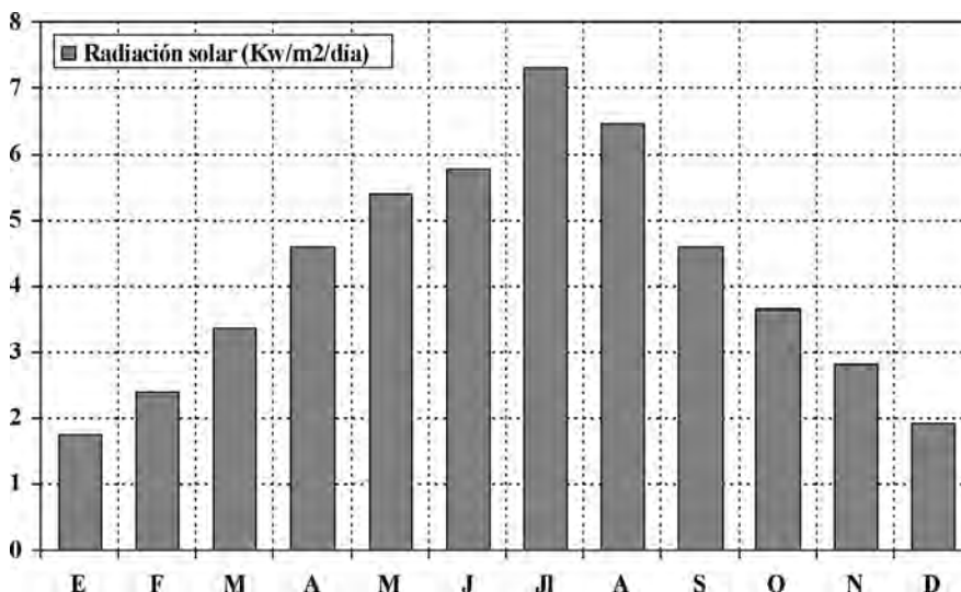
FIGURA 2. Régimen anual de la radiación solar (KW/m 2 /h/diario) en el campus universitario, Universitat Jaume I de Castellón (2003-2010).
