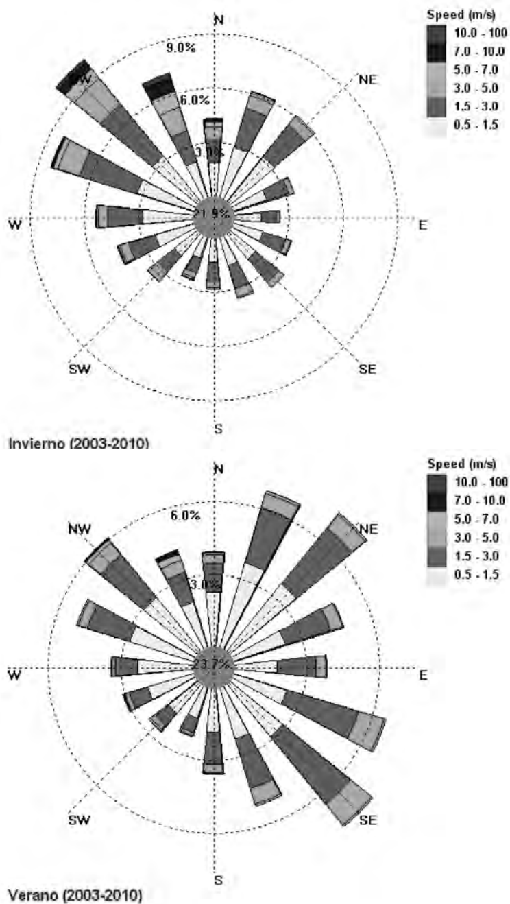
FIGURA 11. Las rosas de vientos (2003-2010) muestran un acusado contraste estacional acorde con el régimen de brisas predominante.
