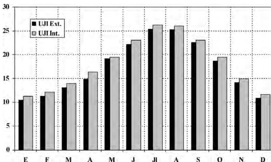
FIGURA 5. Evolución de la temperatura media a lo largo del trienio 2006-2010 en el observatorio de la Facultad de Humanas y en el Observatorio exterior del campus.
