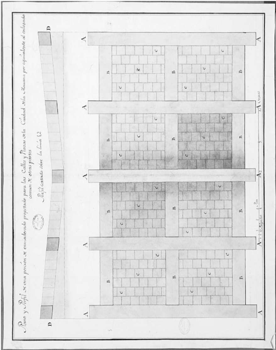
FIGURA 4. Plano y perfil de una porción de enmaderado, proyectado para las calles y plazas de la ciudad de La Habana, por equivalente al enlosado común de otras partes, AGI, MP, Santo Domingo, n° 383
