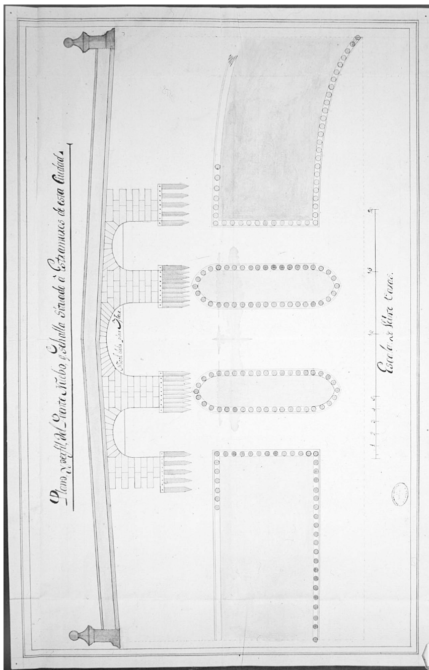
FIGURA 5. Plano y perfil del Puente Nuevo que se halla situado a extramuros de la ciudad [de La Habana]. AGI, MP, Santo Domingo, n° 575.
