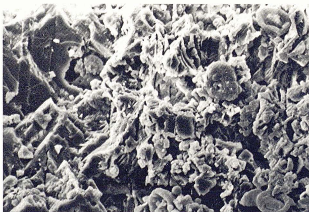
Figura 5: a) Fotografies al microscopi electrònic on s'observa l'increment de superfície deguda a l'acció biològica (RK). Escales gràfiques: 100μm i 20μm. b) Detall de la superfície polida a la mostra RP, on s'observa una certa irregularitat que pot ser l'origen d'una petita quantitat de carbonats particulats. Escales gràfiques: 100μm i 10μm.
