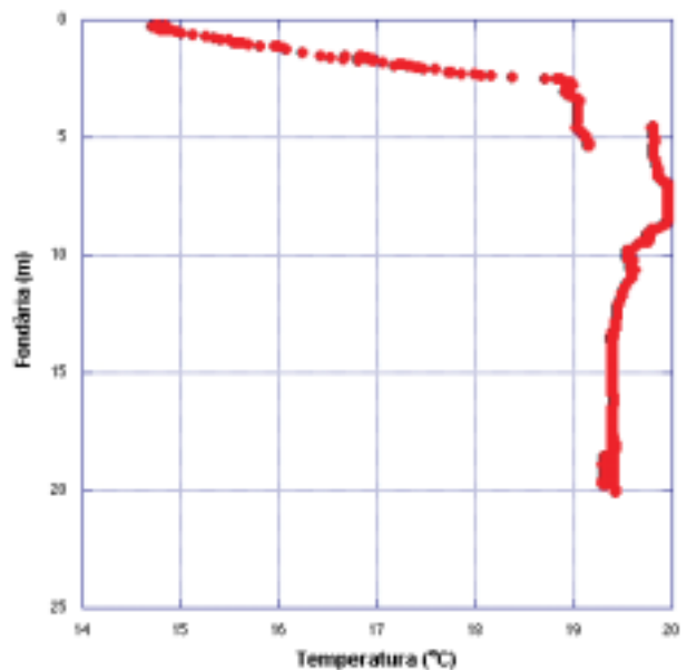
Figura 9: Perfil integrat de temperatura de l'aigua corresponent a la sala d'Entrada i la galeria Esfondrada. Es distingeix una termoclina acusada entre la superfície i els 3 m de fondària, quan la temperatura de l'aigua s'estabilitza i es manté entre 19 i 20° C fins el fons de la cavitat. Es produeix una estratificació inversa, amb l'aigua més calenta ocupant les capes fones i la freda les superficials, tan característica dels llacs anquihalins.
