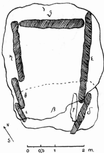
Fig. 17. — Dolmen de la Sureda (Palau Sabardera)
