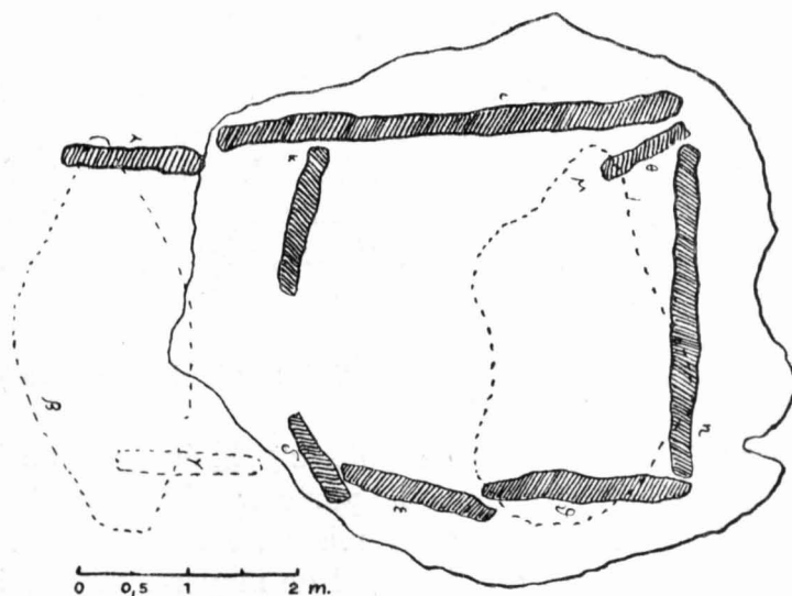
Fig. 19. — Dolmen de la Creu d'en Cobertella (Rosas).
