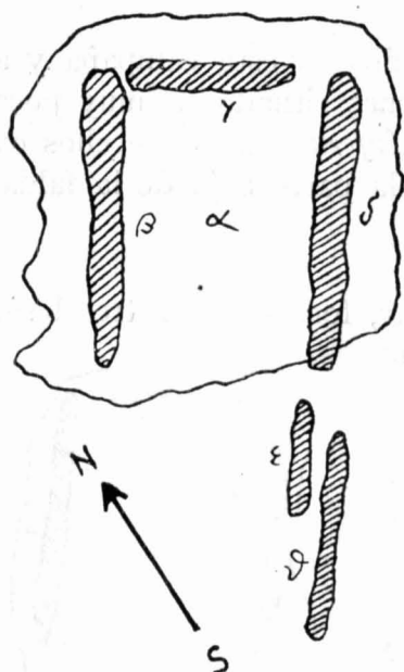
Fig. 2. — Dolmen de la Talaia (Vilajuiga). Escala 1 : 50.
