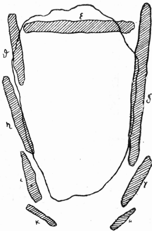
Fig. 14. — Devesa (Pau). Escala 1 : 50.
