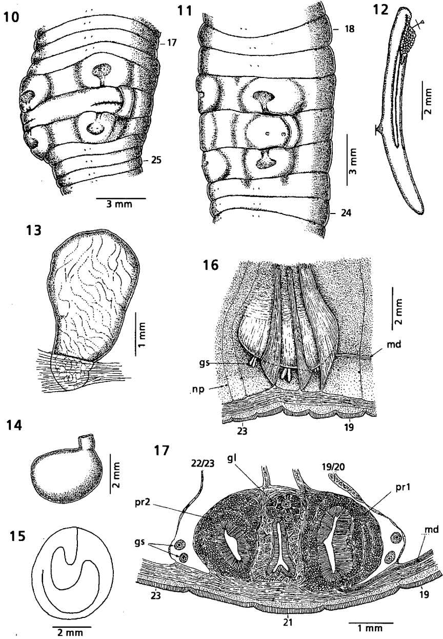
Rhinodrilus appuni pavoni n. subsp.: 10, 11. Vista ventro-lateral de dos especímenes, segmentos XVII-XXV y XVIII-XXIV; 12. Nefridio post-clitelar; 13. Espermateca de 7/8; 14. Glándula calcífera del segmento VII; 15. Corte transversal del intestino en el medio del cuerpo; 16. Vista interna de la parte final derecha masculina, segmentos XIX-XXIII; 17. Corte sagital de la misma: gl. Glándulas asociadas con folículos de las cerdas genitales; gs. Cerdas genitales; md. Conductos masculinos; np. Nefridioporo; pr1, pr2. Primera y segunda glándulas prostatoides; 19/20, 22/23. Septos.
