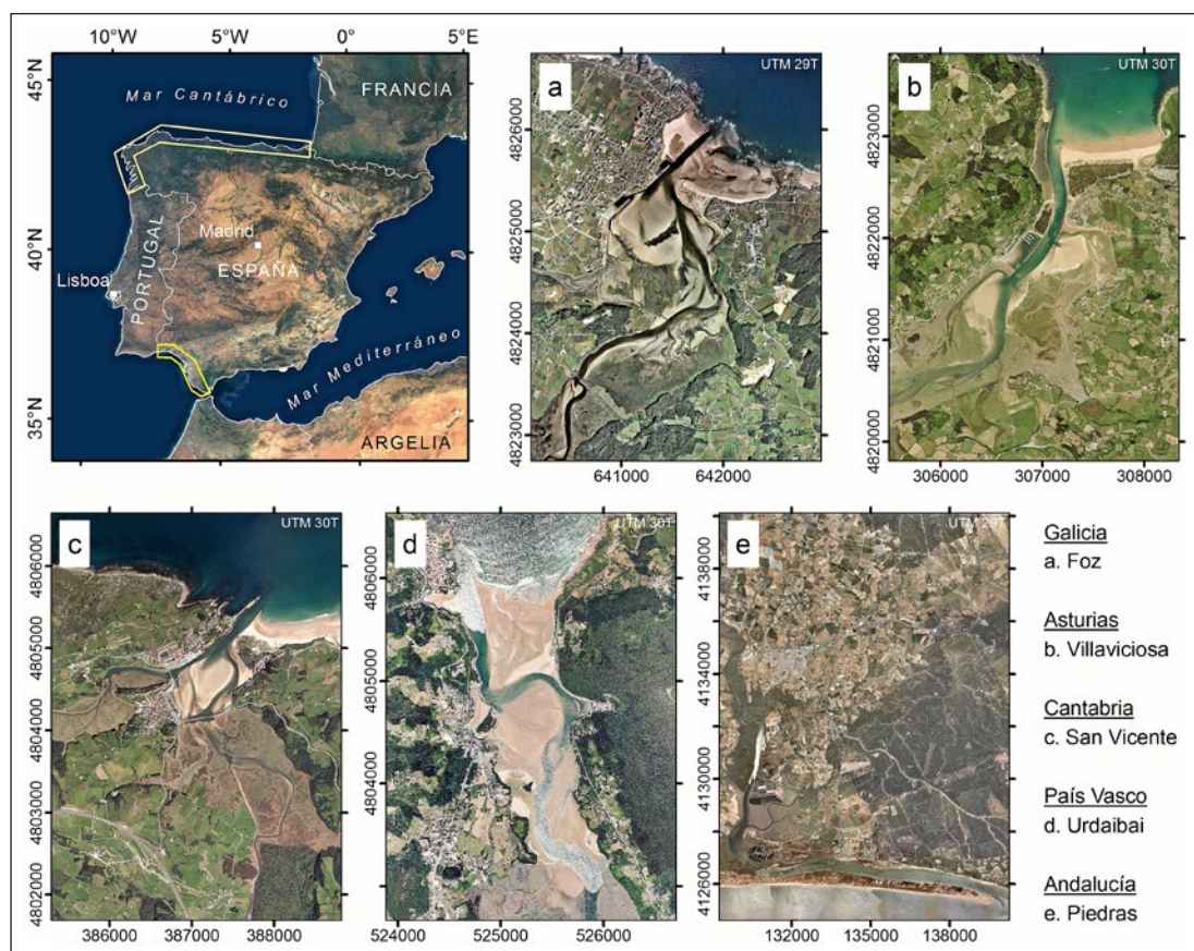
Fig. 1. Sector de costa española donde se desarrollan estuarios y rías, mostrando un estuario característico de cada Comunidad Autónoma: a) Foz (Galicia), b) Villaviciosa (P. Asturias), c) San Vicente de la Barquera (Cantabria), d) Urdaibai (País Vasco), e) Piedras (Andalucía).
