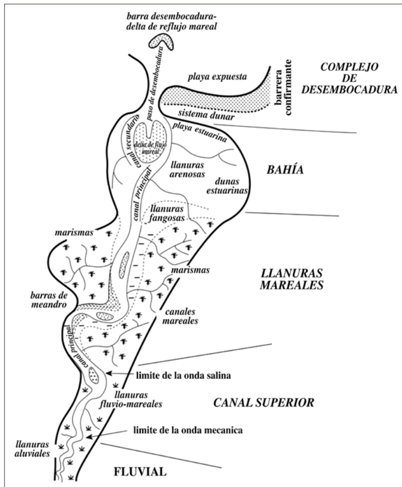
Fig. 2. Modelo de zonación geomorfológica longitudinal de estuarios barrera en costas mesomareales, incluyendo las unidades morfosedimentarias y dinámicas más relevantes (sin escala).
