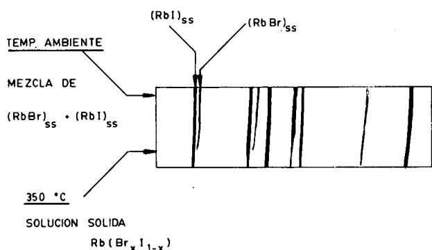
Figura 1. — Diagrama Guinier-Lenné correspondiente a una mezcla binaria de composición 0.7RbI+0.3RbBr. Condiciones experimentales: radiación \text{CuK}\alpha_1 ; monocromador curvo de cuarzo; 40 KV, 16 mA; tiempo de exposición 30 horas; velocidad de desplazamiento de la cámara 1 mm/hora.
