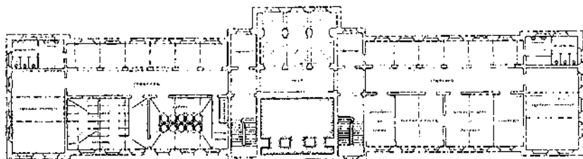
PLANTA DE SEMI-SÒTANS
