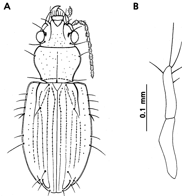
Fig. 1. Tasmanitachoides glabellus n. sp.: A. Habitus, length 2.5 mm; B. ♀ left stylomeres 1 & 2, ventral view.
