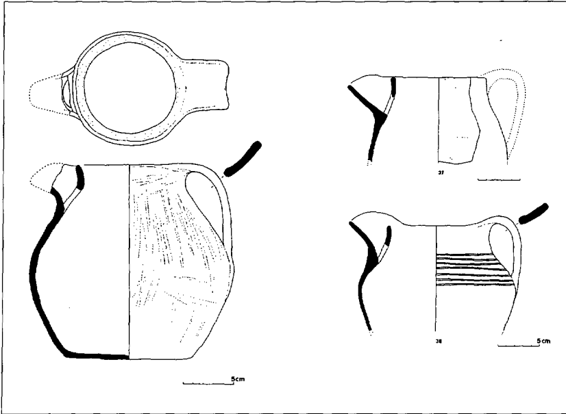
Figura 3.- Sitra espatulada i dues sitres sense espatular, procedents del jaciment de l'Avinguda de la Catedral (Barcelona, Barcelonès)(Dibuix J. ROIG i BUXÓ, 1994).
