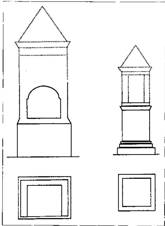
Figura 1. Restitució hipotètica proposada per Von Hesberg (1985) de la Torratxa (Vilablareix) (esquerra) i la Torre del Moro (Lloret de Mar) (dreta).
