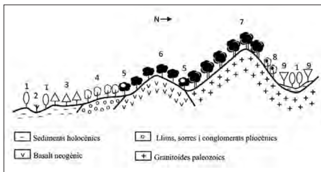
Figura 1. Transsecte esquematitzat de la vegetació potencial de la plana de la Selva. 1. verneda amb rèvola ( Lamio-Alnetum glutinosae subass. stellarietosum holosteae ); 2. salzedra de sargues ( Saponario-Salicetum purpureae ); 3. freixeneda de freixe de fulla petita amb roure martinenc ( Carici-Fraxinetum oxycarpae subass. quercetosum pubescentis ); 4. roureda calcifuga de roure martinenc ( Carici-Quercetum canariensis subass. holcetosum mollis ); 5. bosc mixt d'alzina i roure martinenc ( Viburno-Quercetum ilicis subass. quercetosum pubescentis ); 6. alzinar amb marfull ( Viburno-Quercetum ilicis subass. pistacietosum ); 7. sureda ( Viburno-Quercetum ilicis subass. quercetosum suberis ); 8. freixeneda de freixe de fulla petita i roure pènel ( Carici-Fraxinetum oxycarpae subass. quercetosum roboris ); 9. roureda de roure africà típica ( Carici-Quercetum canariensis subass. quercetosum canariensis ).
