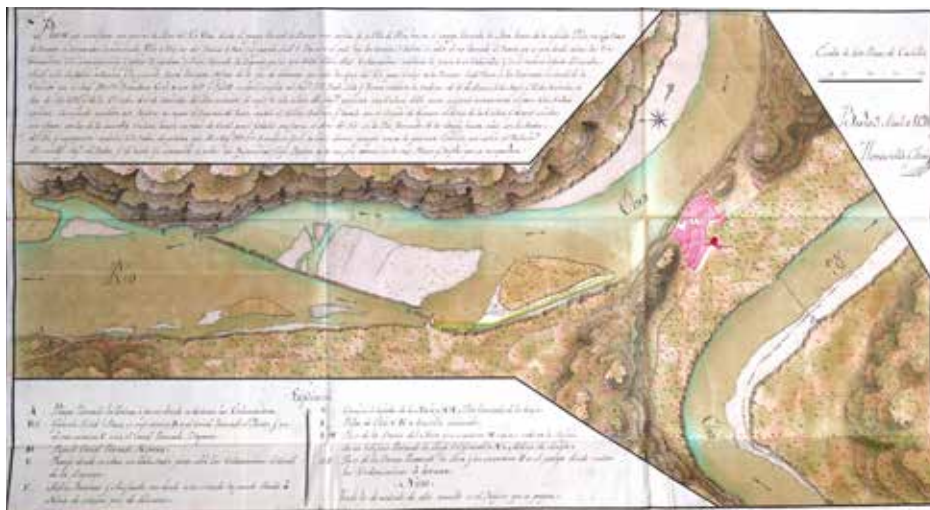
Figura 1. Plano general del proyecto del azud de Flix
