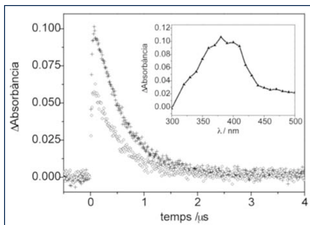
Figura 7. Decaiments temporals de la ^3\text{BM-DBM(K)-Me} monitorats a 380 nm en absència de filtre (creus) i en presència del filtre 2 (rombes buits) en una proporció 1:1 pes/pes. Requadre: Espectre d'absorció triplet-triplet de l'avobenzona metilada en acetonitril i sota atmosfera inert.
