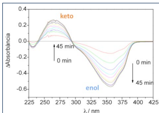
Figura 5. Espectres d'absorció diferència de l'avobenzona irradiada en acetonitril. Cada traça correspon a la diferència entre l'espectre de la mostra irradiada i l'inicial sense irradiar. La irradiació s'ha dut a terme periòdicament, durant 45 minuts.
