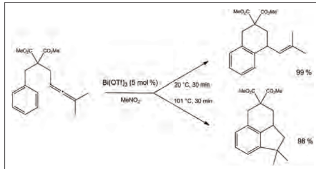
FIGURA 10. Hidroarilació d'al-lens i doble ciclació.
