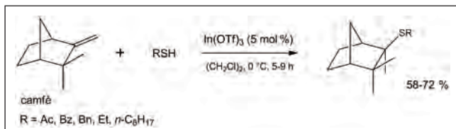
FIGURA 3. Síntesi de derivats del camfè.
