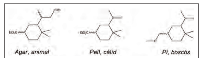
FIGURA 7. Avaluació olfactiva d'estructures de tipus gem -dimetilciclohexà.
