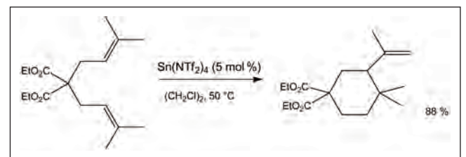
FIGURA 5. Exemple de ciclació d'un diè-1,6.
