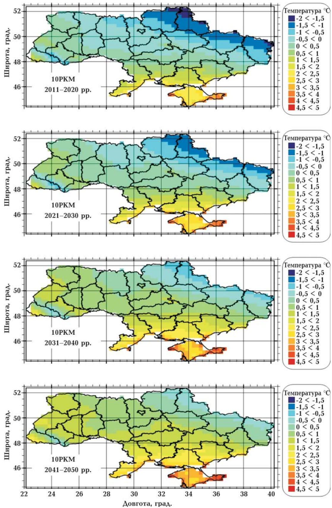
Рис. 4. Проекції середньої температури опалювального періоду (°C) по десятиріччях до середини ХХІ ст.
