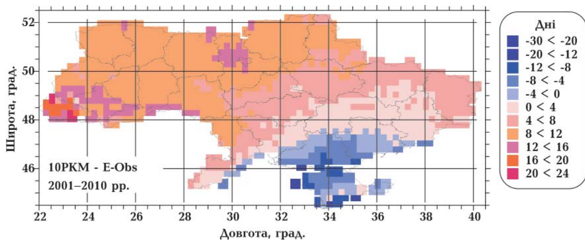
Рис. 2. Різниці (похибки) між даними ансамблю 10 РКМ та E-Obs щодо тривалості опалювального сезону (дні) у базовий період 2001—2010 рр.
