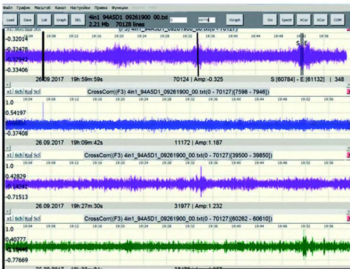
Рис. 6. Запис 1-ї години запису до і на початку вибухів (Калинівка, 26 вересня, 19:00 UTC, верхній графік) і корелограми (внизу) за відсутності імпульсних сеймопакетів (тільки шум) і наявності двох слабких сейсмічних сигналів.
