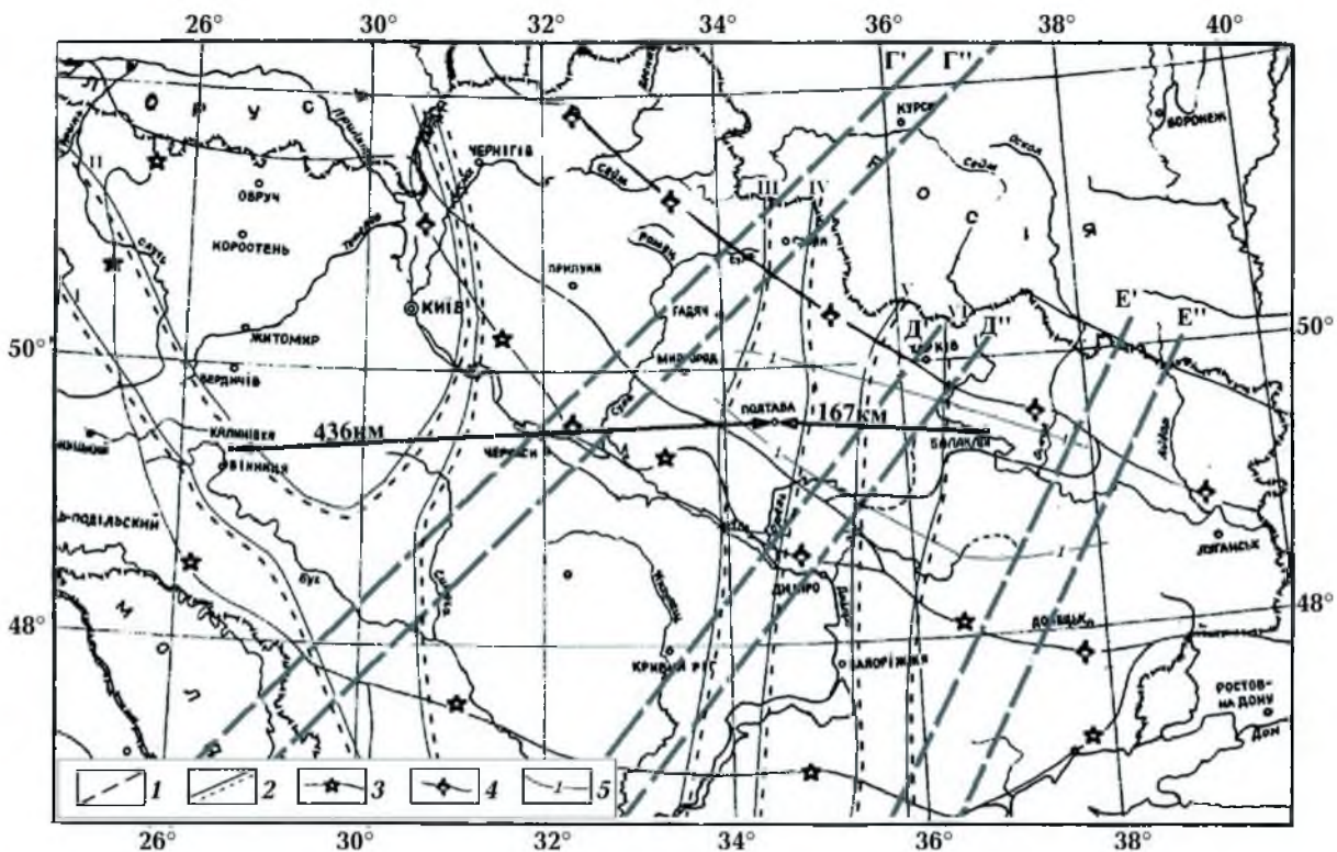
Рис. 3. Карта території досліджень з елементами блокової геотектоніки України і трасами сейсмічних сигналів: 1 — мантійні розломи ( \Gamma' — \Gamma'' , Д' — Д'' і Е' — Е'' ); 2 — глибинні розломи; 3 — межа Українського щита; 4 — межа Дніпровсько-Донецької западини; 5 — міжблокові розломи [Сологуб, 1986].
