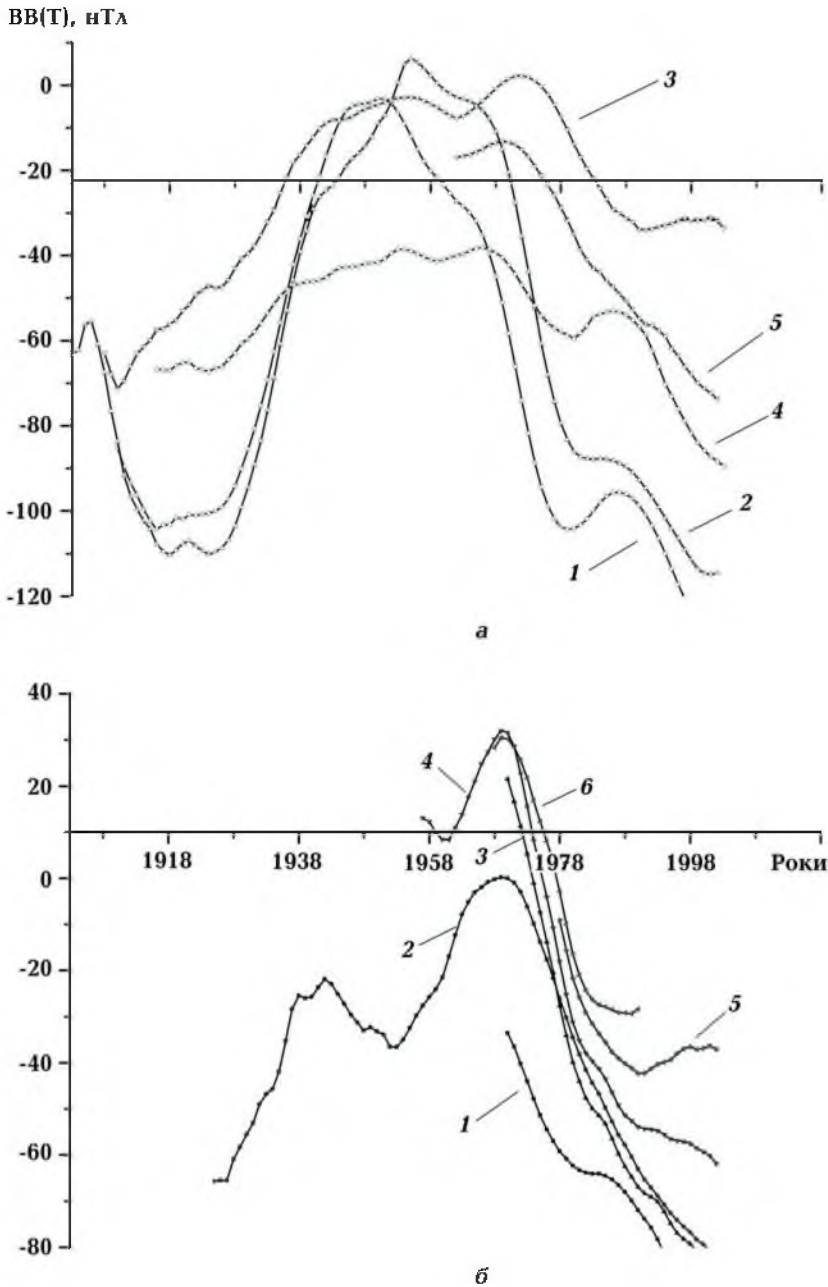
Рис. 5. Зміни ВВ(Т) на магнітних обсерваторіях, розміщених на Північній Америці: а — східне Американське узбережжя (1 — Фредеріксбург (FRD), 2 — Аженкурт (AGN), 3 — Сітка (SIT), 4 — Таксон (TUC), 5 — Вікторія (VIC)); б — різні широти (1 — Боулдер (BOU, \varphi = 40^\circ ), 2 — Мінук (MEA, \varphi = 54^\circ ), 3 — Форт Черчилл (FCC, \varphi = 59^\circ ), 4 — Бейкер Лейк (BLC, \varphi = 40^\circ ), 5 — Кермідж Бей (CBV, \varphi = 69^\circ ), 6 — Моулд Бей (MBC, \varphi = 76^\circ )).
