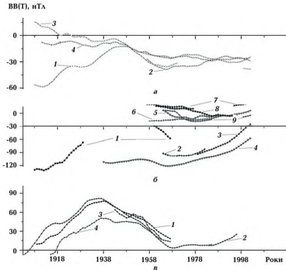
Рис. 4. Величини ВВ(Т) на обсерваторіях: а — на ТО-плиті (1 — Гонулулу (HON)) і на межі ТО-плити з ІА-плитою (2 — Макуорі (MCQ), 3 — Амберлі (AML), 4 — Апія (API)); б — на Африканській тектонічній плиті на обсерваторіях Східної Африки (1 — Тананаріве (TAN), 2 — Мапуту (LMM), 3 — Хартебесток (HBK), 4 — Херманус (HER), 5 — Адіс-Абеба (AAE)) та Західної Африки (6 — М'Бур (MBO), 7 — Таманрассет (TAM), 8 — Бангуї (BNG), 9 — Гуйнар (GUI)); в — єгипетській (1 — Хелвен-Міссалат (HLW-MLT)), грузинській (2 — Тбілісі (TFS)), ліванській (3 — Ксара (KSA)), російській (4 — Казань (KZN)).
