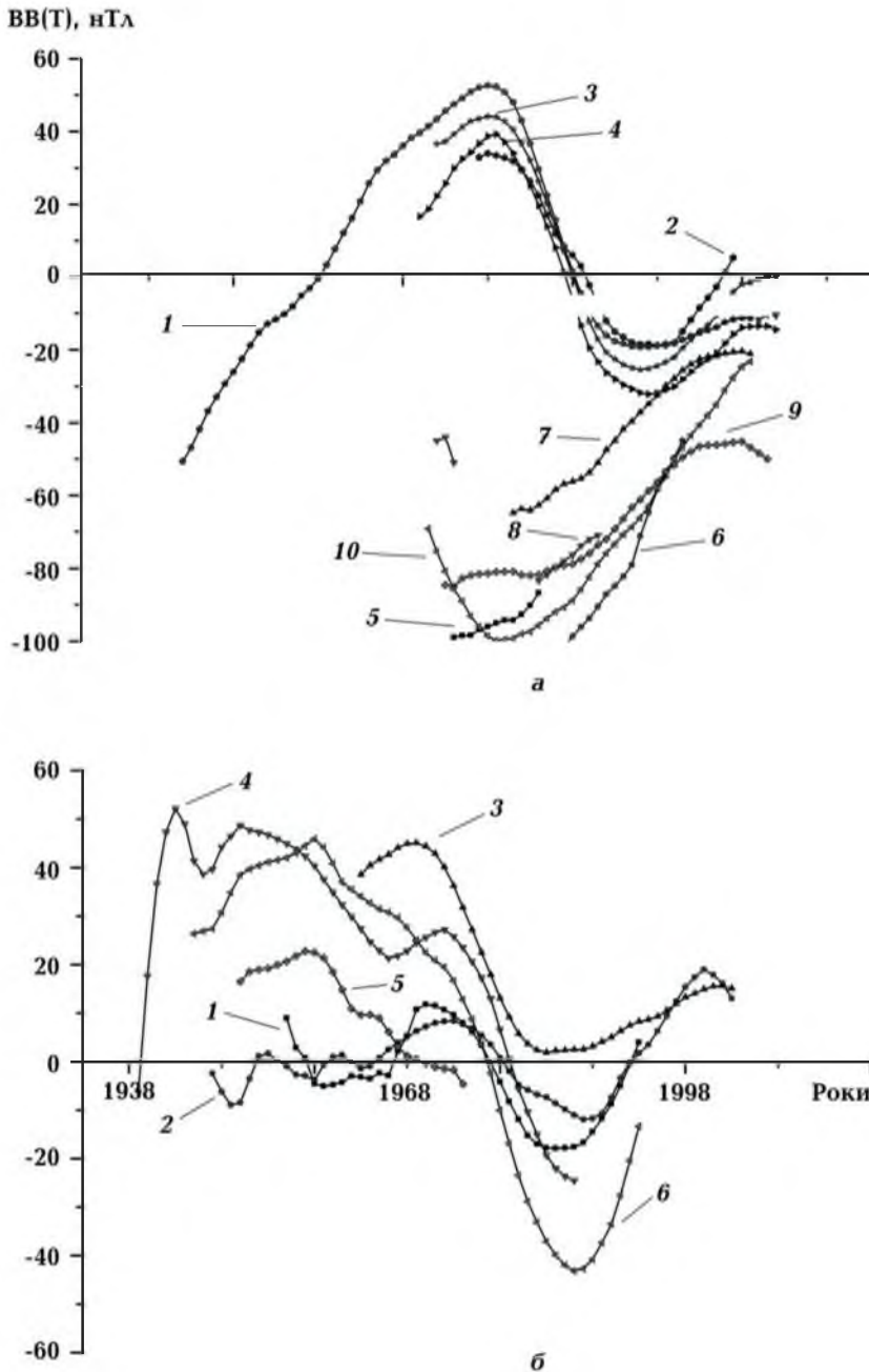
Рис. 8. Зміни ВВ(Т) у високих широтах Північної та Південної півкуль: a — полярна шапка Північної півкуль (обсерваторії: 1 — Годхавн (GDH) ( \varphi = 69^\circ , \lambda = 306^\circ\text{E} ), 2 — Туле (THU), 3 — Алерт (ALE), 4 — Резольют Бей (RES); високі широти Південної півкуль (5 — Восток (VOS), 6 — Молодьожная (MOL), 7 — Дьбюмон-д-Юр-віль (DRV), 8 — Мирний (MIR), 9 — Скот Бейс (SBA), 10 — Маусон (MAW)); б — авроральна зона Північної півкуль (обсерваторії: канадські (1 — Барров (BRW), 2 — Коледж (СМО)), ірландська (3 — Лейрвокур (LVR)); російські (4 — ДІК, 5 — ТІК, 6 — ССС)).
