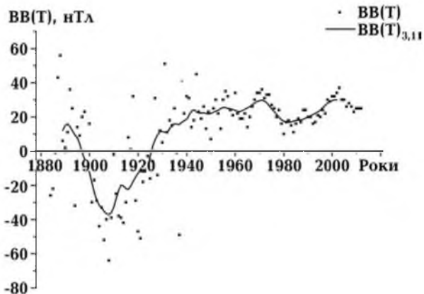
Рис. 2. Вікові варіації напруженості геомагнітного поля, згладжені 3- та 11-річними біжними вікнами ВВ(T) 3,11 , та незгладжені величини ВВ(T) на французькій магнітній обсерваторії Шамбон-ла-Форе (CLF).
