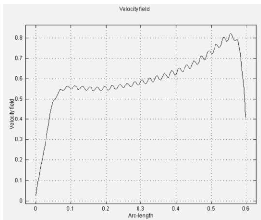
Рисунок 4 –Графіки зміни швидкості повітря до проходження ним випарника
