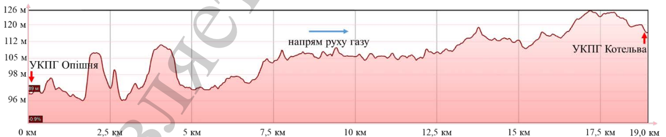
Рис. 5. План-профіль траси низьконапірного газопроводу УКПГ Опішня – УКПГ Котельва (ділянка № 5)
