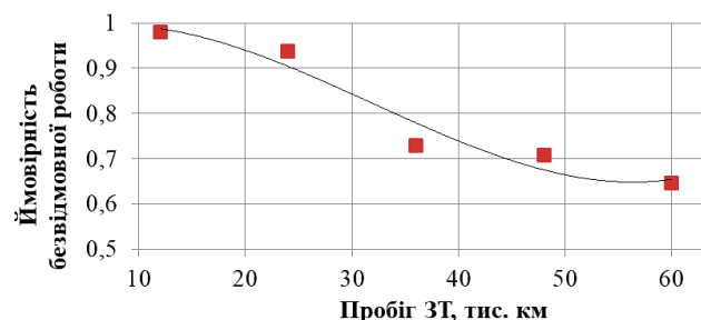
Рис. 3. Зміна ймовірності безвідмовної роботи коробки переключення передач від пробігу ЗТ
