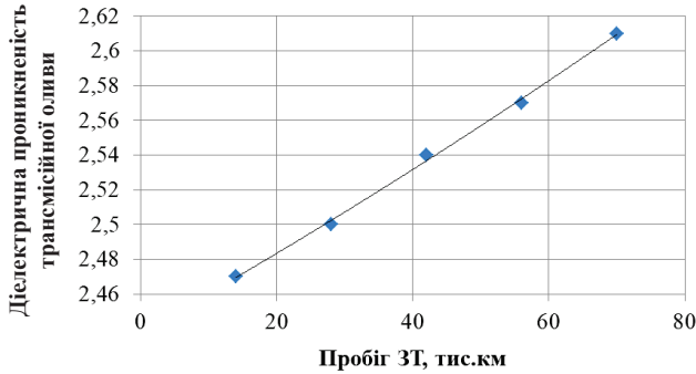
Рис. 6. Зміна середніх значень діелектричної проникненості трансмісійної оливи від пробігу засобу транспорту
