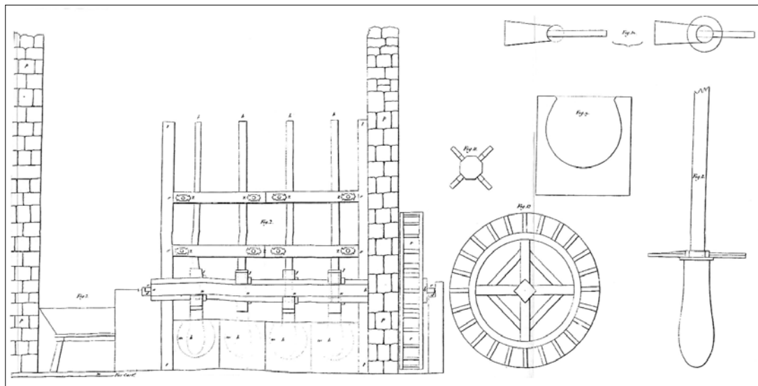
Plànol horitzontal d'un dels molins de Manresa (Arte de fabricar el salitre y la pólvora. 1833)
