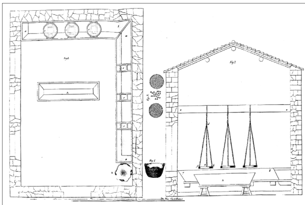
"Oficina del graneador". (Arte de fabricar el salitre y la pólvora. 1833)
