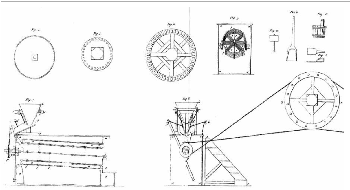
"Pulverización del salitre y el azufre" (Arte de fabricar el salitre y la pólvora. 1833)
