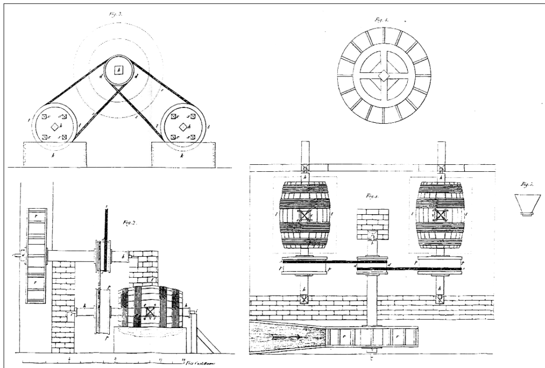
"Plano de perfil y corte de la maquina destinada a pavonear la pólvora" (Arte de fabricar el salitre y la pólvora. 1833)
