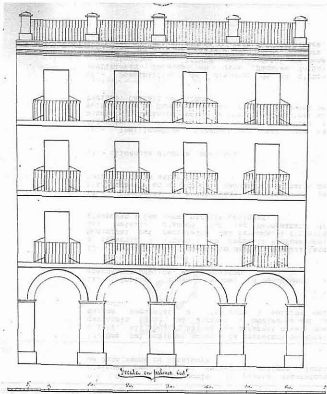
Alçat adjuntat a la sol·licitud d'obres presentada l'any 1864.
