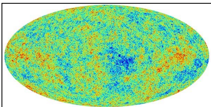
Figura 2. Mapa del cel mostrant el fons còsmic de microones tal com l'ha observat el satèl·lit Planck de l'Agència Espacial Europea. La imatge mostra la temperatura de la radiació observada, les variacions que s'observen són corresponen a una part entre 100.000. Aquestes mesures certifiquen fins a quin punt el nostre Univers és homogeni quan l'observem a gran escala. Crèdits: ESA
