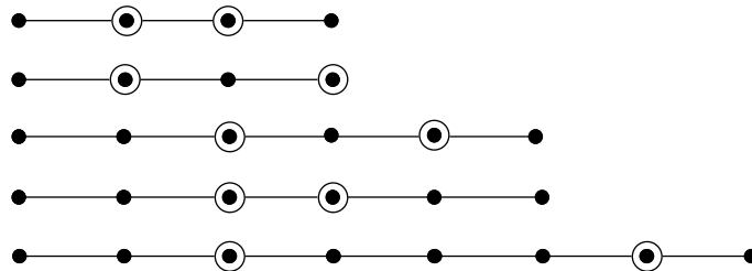
FIGURA 7: Exemples de conjunts k -distància dominadors. Als dos primers grafs s'han assenyalat dos conjunts 1-distància dominadors minimal, mentre que al tercer, quart i cinquè s'illustren conjunts 2-distància dominadors minimal. Com es pot observar la distància entre els vèrtexs d'aquests conjunts pot ser més gran o igual a 1 en els dos primers casos i més gran, igual o menor a 2 en els tres últims.
