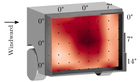
(b) Optimised flap angles (0°,0°,0°,0°,0°,7°,0°,7°,14°)
