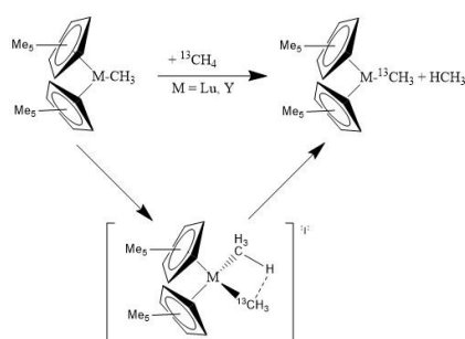
Figura 5: Reacción a través del mecanismo metátesis de enlace sigma
