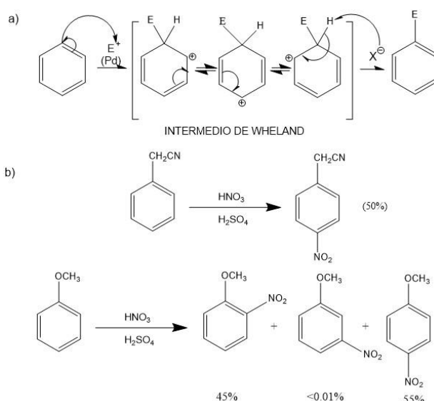
Figura 12: a) Mecanismo general de la S_EAr e intermedio de Wheland. b) Ejemplo S_EAr orientación orto y para.
