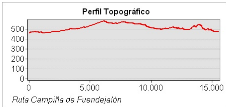
Gráfico perfil topográfico Viñedos Centenarios
