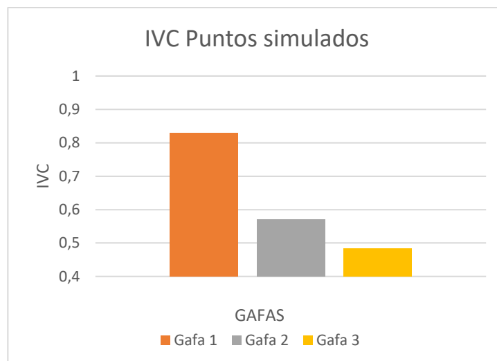
Figura 22. Gráficas IVC datos simulados. Optotipo puntos
