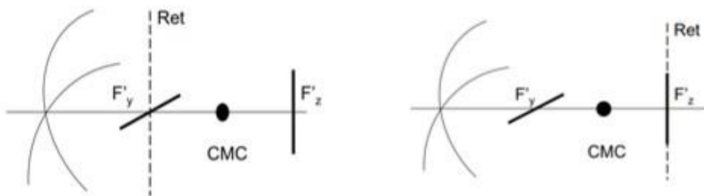
Figura 5.A. Astigmatismo hipermetrope simple. Figura 5.B. Astigmatismo miope simple (17)
