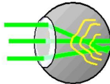
Figura 1.B. Frente de onda aberrado
