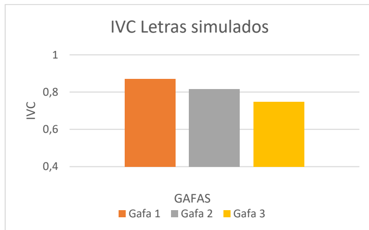
Figura 21. Gráficas IVC datos simulados. Optotipo letras
