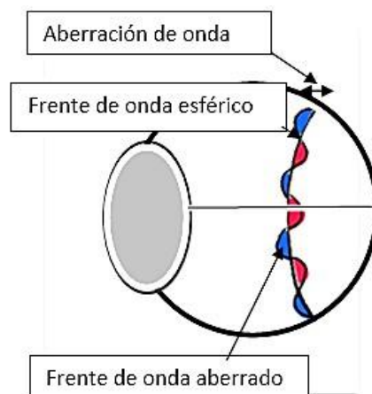
Figura 2. Aberración de frente de onda
