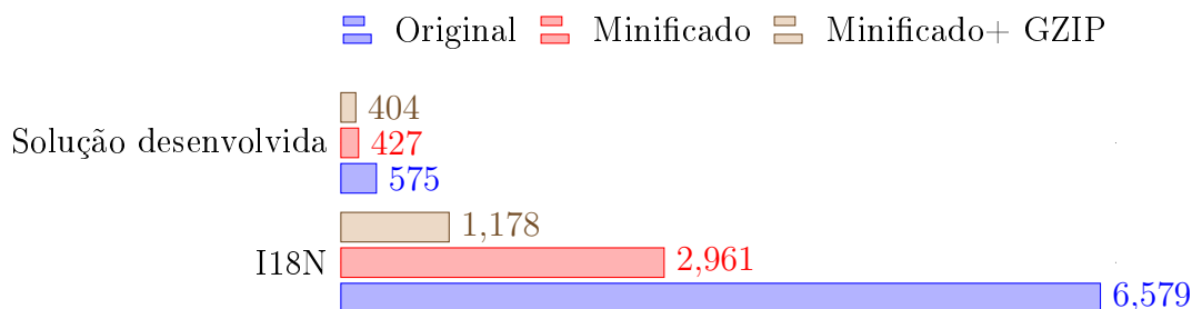
Figura 3.3: Gráfico com comparação do tamanho entre versões (em Bytes)
