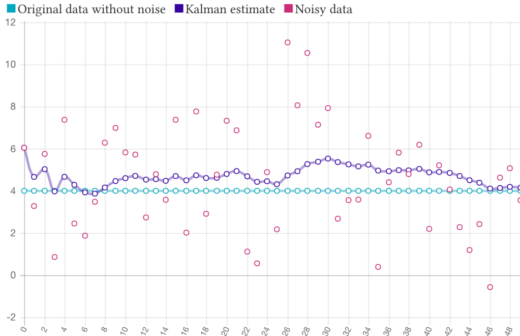
Figura 3.15: Exemplo da aplicação do Filtro Kalman [5]
