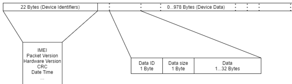
Figura 3.10: Estrutura do Pacote NB-IOT
