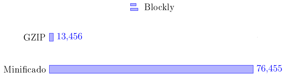
Figura 3.9: Gráfico com comparação do tamanho do plugin Blockly (em Bytes)
