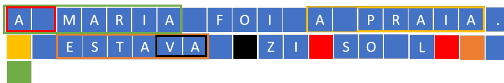
Figura 2.8: Sequência comprimida com LZ77(palavras e sequências)
