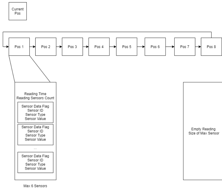
Figura 3.12: Array Circular com leituras
