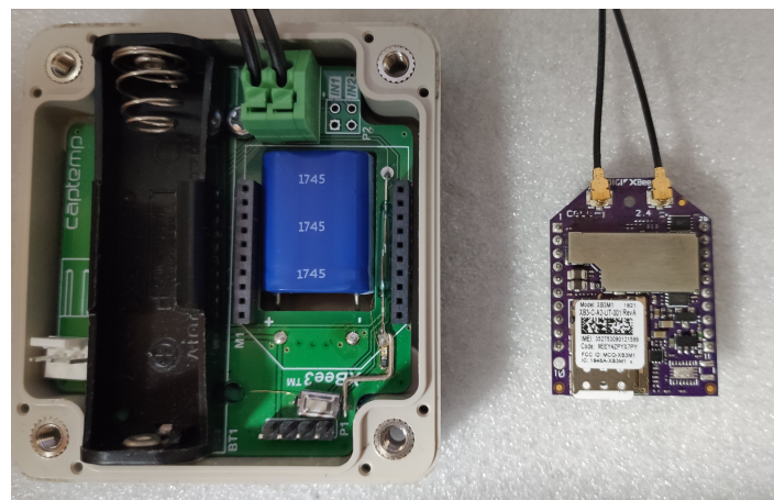
Figura 2.2: Módulo Xbee 3 e placa de expansão desenvolvida pela Captemp
