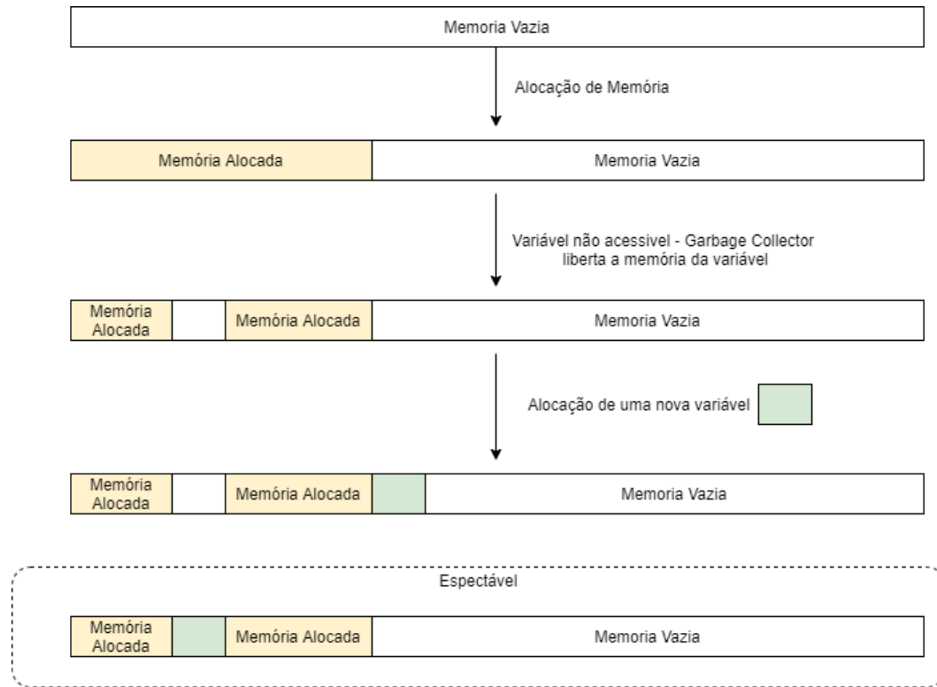
Figura 3.11: Comportamento da gestão de Memória do MicroPython
