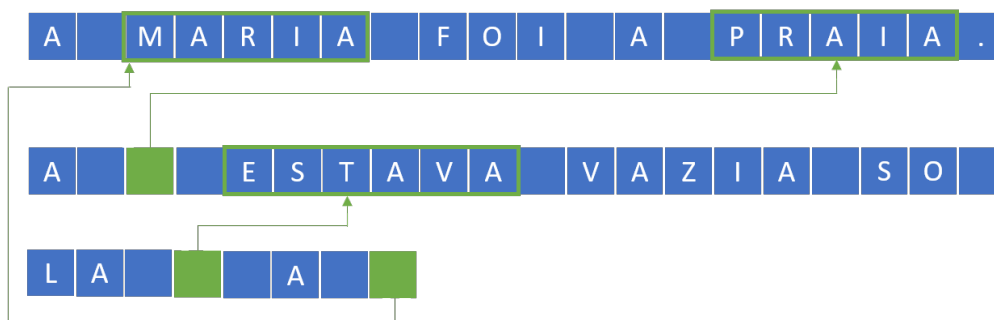
Figura 2.7: Sequência comprimida com LZ77 (apenas palavras)
