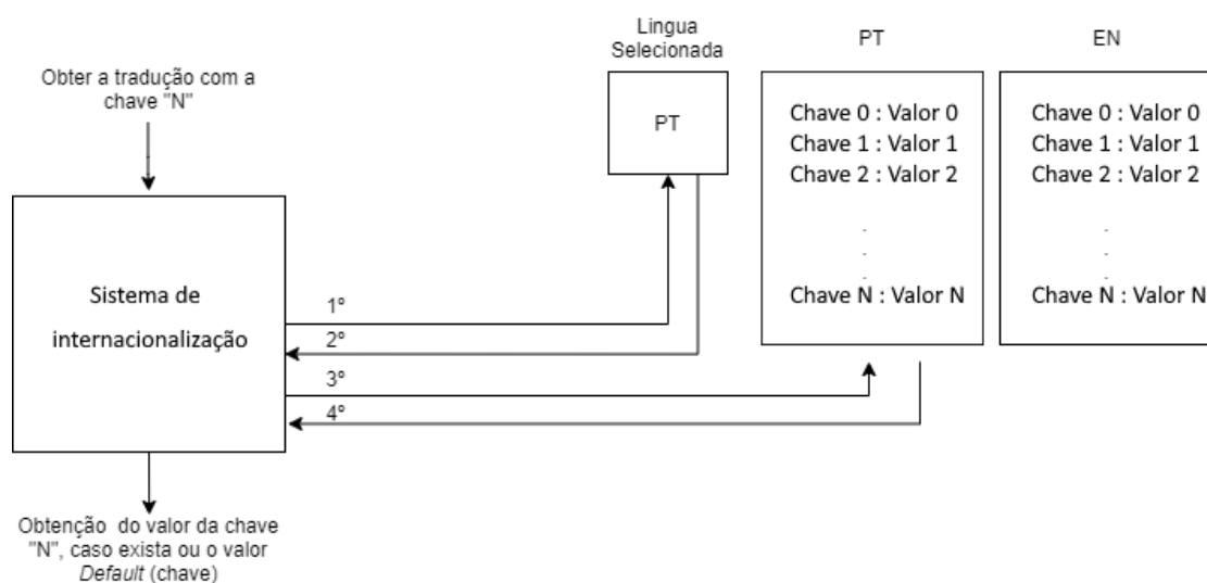
Figura 3.1: Processo da obtenção da tradução de um valor
