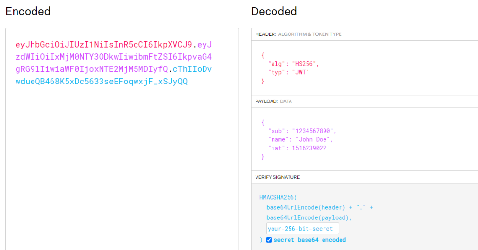
Figura 3.13: Token JWT codificado e decodificado [4]
