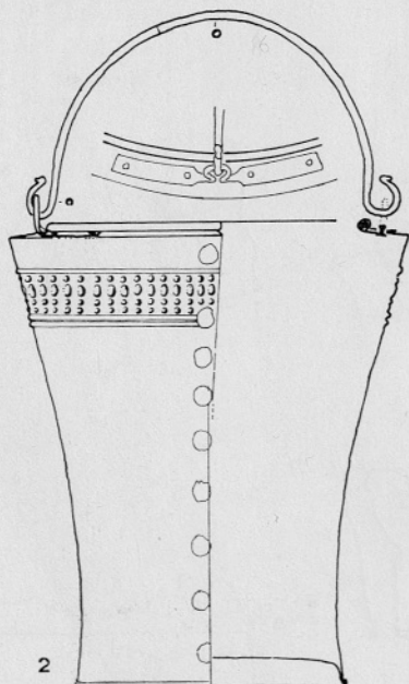
Valična vas. Bron. Po F. Staretu, Zbornik fil. fak. Ljubljana 2 (1955) T. 15, 17 Valična vas. Bronze. Nach F. Starè Zbornik fil. fak. Ljubljana 2 (1955) T. 15, 17
