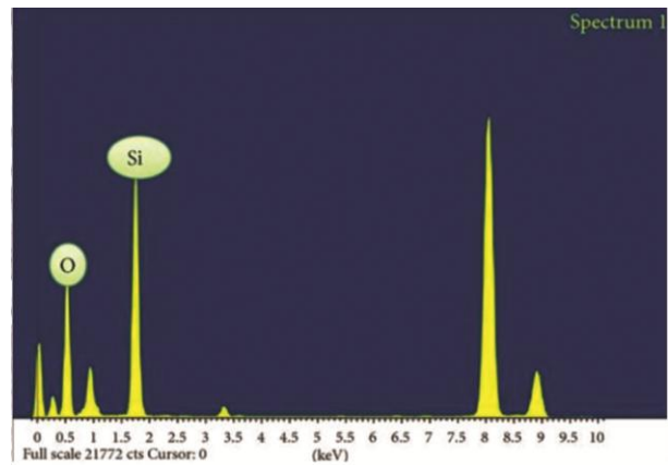
Fig. 6 — EDS spectra
