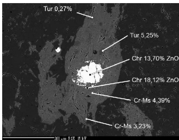
Obr. 1 Reliktne zrnó chromitu bohatého na Zn (biely) obklopené aureolou Cr-muskovitu (svetlošedá) so stĺpkami Cr-turmalínu (stredná šedá) v kremeni (čierna) v odrazených elektrónoch (BEI). Čísla bez označenia sú obsahy Cr_2O_3 . Vzorka QTTR-4, Nitra, Malá Skalka.
