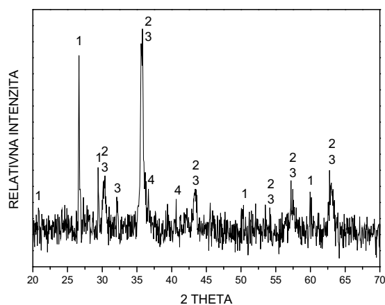
Obr. 1 RTG záznam lúženca (1 – kremeň, 2 – chromit, 3 – magnetit, 4 – wüstit)
