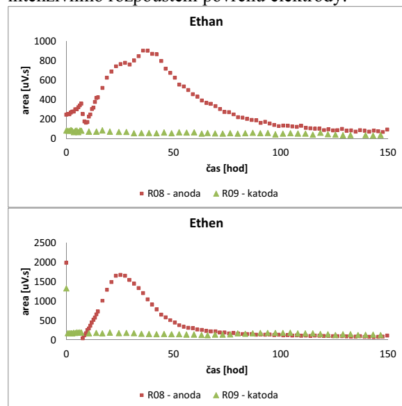
Obr. 5 Vývin rozkladných produktů dechlorace CIE v reaktoru
