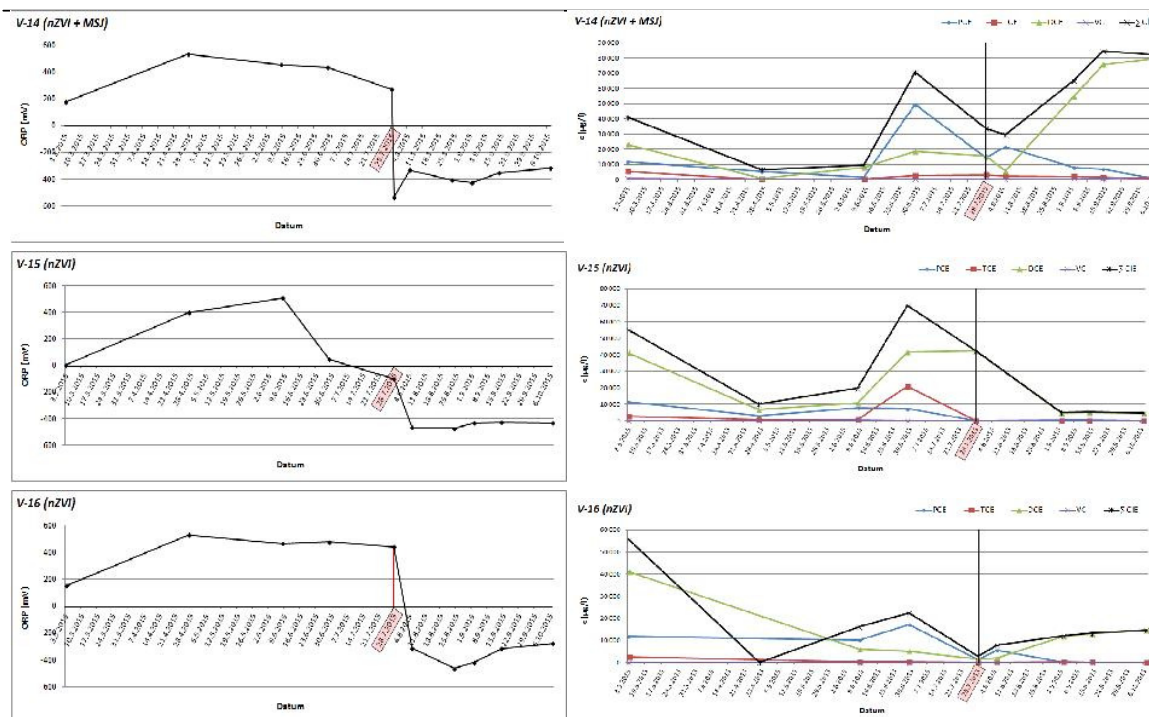
Obr. 4 Vývoj ORP(levý sloupec) a jednotlivých CIE(pravý sloupec) v aplikačních vrtech V11 – V16; lokalita B
