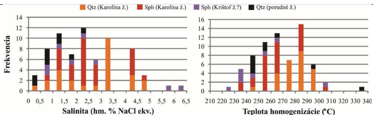
Obr. 3 Histogramy počtosti hodnôt salinit a homogenizačných teplôt fluidných inklúzií.
