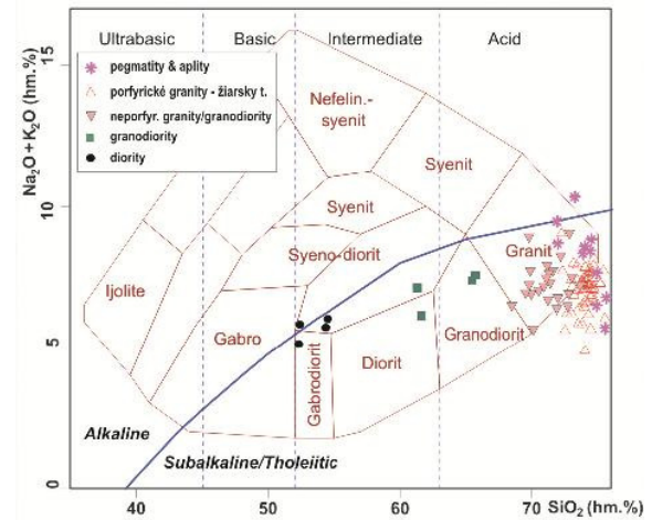
Obr. 2 TAS klasifikačný diagram granitoidov Žiaru.
