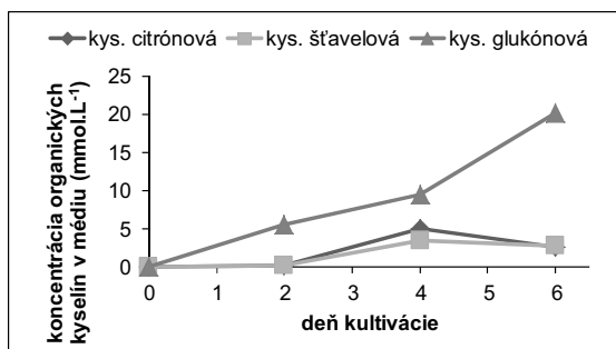
Obr. 3 Obsah organických kyselín v živnom médiu počas 6-dňovej inkubácie mikroskopickej vláknitej huby A. niger
