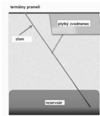
Obr. 1 Jednoduchý koncepčný model pre geotermálny systém
