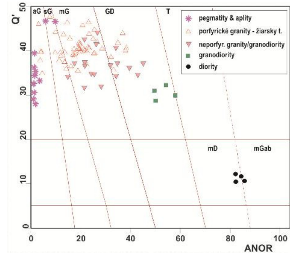
Obr. 3 Diagram Q'-ANOR s využitím mezonormy na detailnejšie odlišenie jednotlivých typov granitoidov.
