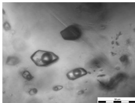
Obr. 1 Koexistencia kvapalno-plynných a plynných inklúzií (var fluíd) v kremeňi rudného štádia Au mineralizácie (žilný typ Agnesa).
