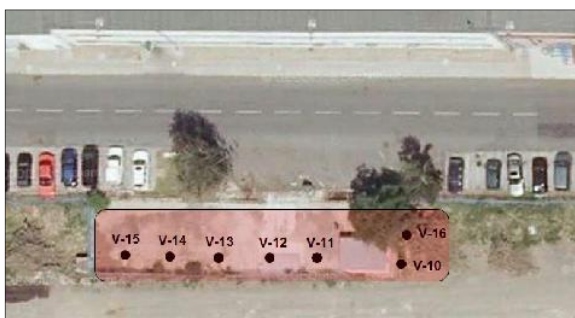
Obr. 2 Lokalita B – sanační oblast s aplikačními vrty V11 – V16
