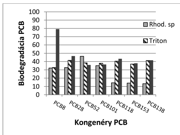
Obr. 2 Biodegradácia jednotlivých kongenéro PCB bakteriálnym kmeňom Rhodococcus sp. bez surfaktantu ( Rhod. sp. ), s prídavkom syntetického surfaktantu (Triton) a biosurfaktantu (Ramnolipid).
