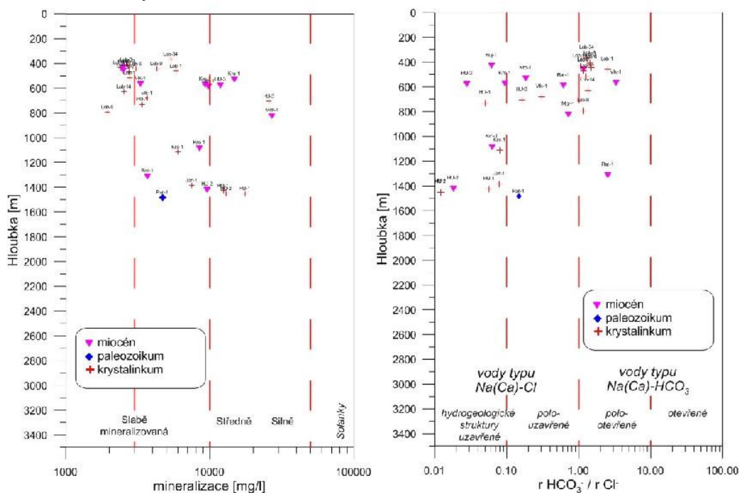
Obr. 2 Celková mineralizace vrstevních voda koeficient r \text{HCO}_3^- / r \text{Cl}^- ve studované oblasti ve vztahu k hloubce uložení kolektoru.
