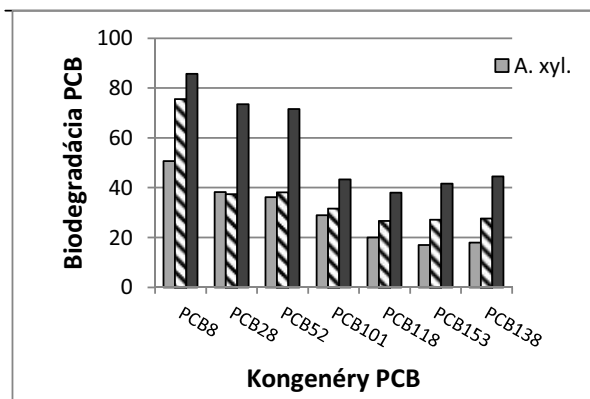
Obr. 1 Biodegradácia jednotlivých kongenéro PCB bakteriálnym kmeňom Achromobacter xylosoxidans bez surfaktantu ( A. xyl. ), s prídavkom syntetického surfaktantu (Triton) a biosurfaktantu (Ramnolipid).
