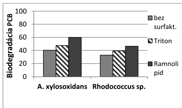
Obr. 3 Biodegradácia celkových kongenéro PCB dvomi bakteriálnymi kmeňmi Achromobacter xylosoxidans a Rhodococcus sp. bez surfaktantu (bez surfakt.), s prídavkom syntetického surfaktantu (Triton) a biosurfaktantu (Ramnolipid).
