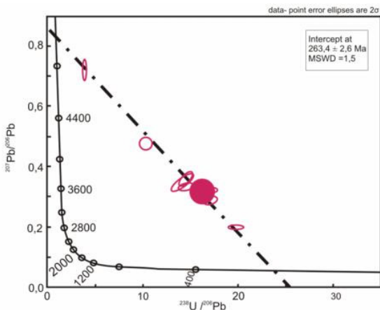
Obr. 8 LA ICP MS veky apatitov
