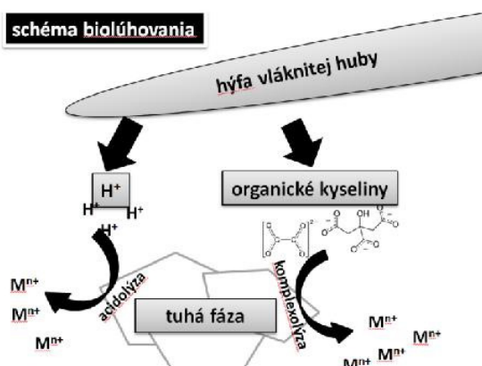
Obr. 1 Schéma uvoľňovania katiónov kovov z povrchov pôdných častíc a minerálov účinkom kyslých vodíkov a organických kyselín produkovaných mikroskopickou vláknitou hubou.
