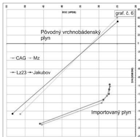
Obr.6: Izotopová charakteristika plynu vrtu MZ a importovaného plynu
