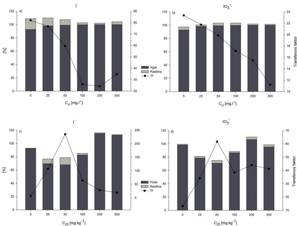
Obr. 2 Obsah extrahovaného jódu z agarového živného média a biomasy (a, b) a z pôdy a biomasy (c, d) s hodnotami transferového faktora (Tf) vo vzťahu k počítateľnej koncentrácii I^- a IO_3^- v rastovom substráte v percentách
