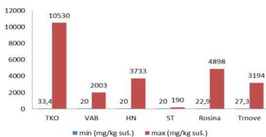
Obr.2: Príklady lokalít s obsahmi bóru typickými pre pozadie (min) a pre zdrojovú oblasť (max) v zemi
