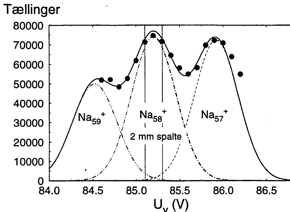
Figur 4.3: Opløsningsevnen af Wienfilteret bestemt eksperimentelt. Sorte cirkler: Målt intensitet af klyngebeamt som funktion af U_v . Den fuldt optrukne linie er summen af de 3 Gausskurver. Gausskurverne er fittet manuelt til at give god overensstemmelse mellem målepunkterne og den fuldt optrukne linie.
