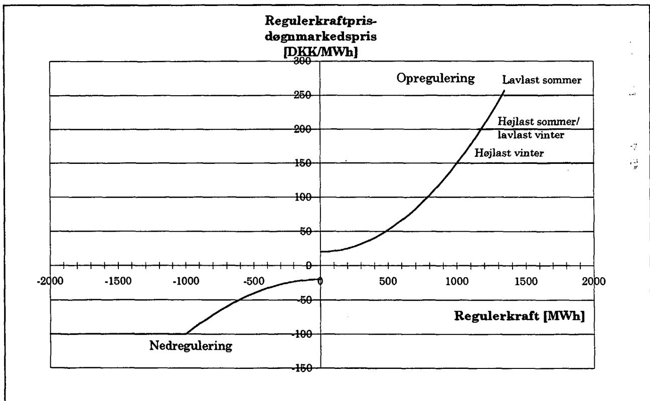
Figur 3-2 Forskellen mellem regulerkraftprisen og døgnmærkedsprisen som funktion af salget af regulerkraft i en given driftstime. Den numeriske værdi af forskellen angiver omkostningerne ved at købe eller sælge en given effekt på elbørsen, og derefter i driftstimen aftage eller levere en anden effekt end den aftalte.
