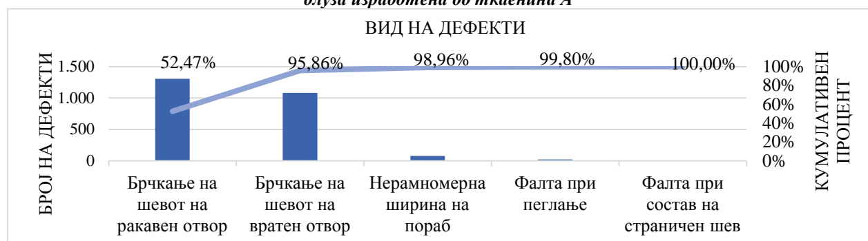
Слика 4. Парето дијаграм на учество на бројот на дефекти во вкупниот број на дефекти кај женска блуза изработена од ткаенина Б
