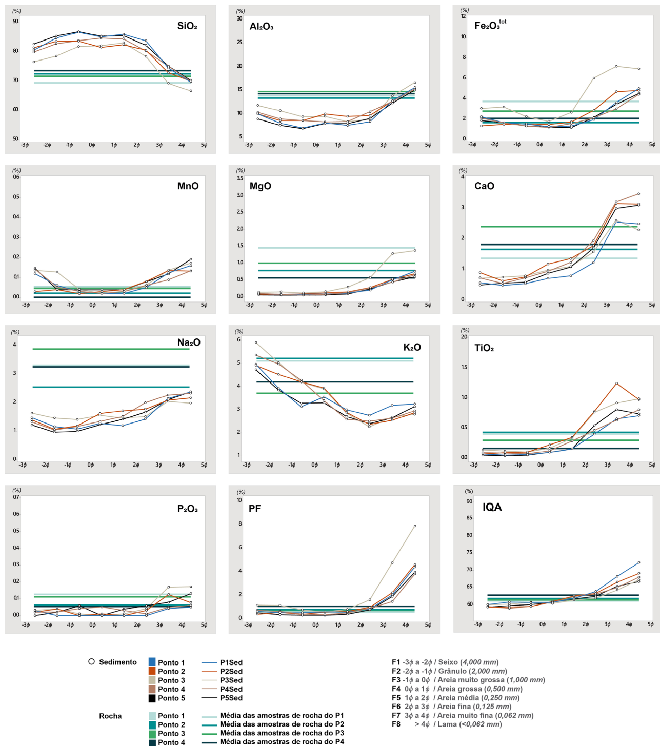
Figura 9. Concentração em (%) de elementos maiores e do Índice Químico de Alteração para as amostras de sedimento versus tamanho de grão expressos em \phi de seixo (-3 \phi a -2 \phi ) a lama (> 4 \phi ), e as concentrações médias das amostras de rocha.
