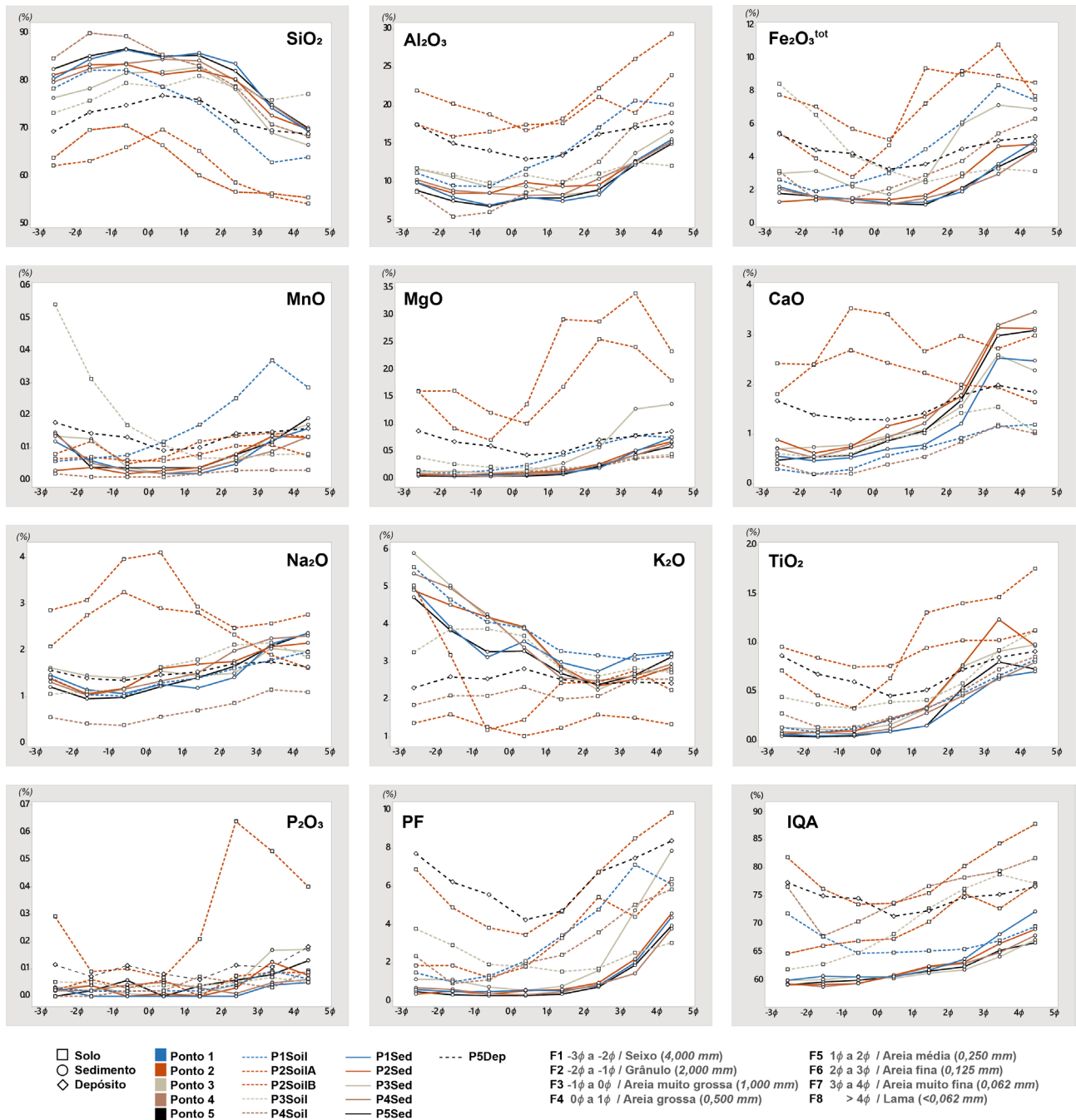
Figura 5. Concentração (%) de elementos maiores e do Índice Químico de Alteração para as amostras de solo, sedimento e depósito versus tamanho de grão. O tamanho de grão é expresso em phi (φ) de seixo (-3 φ a -2 φ) a lama (> 4 φ).
