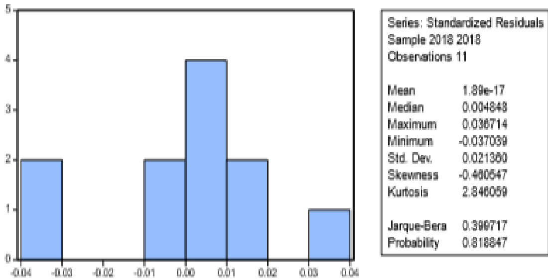
Gambar 4.1 Hasil uji normalitas
