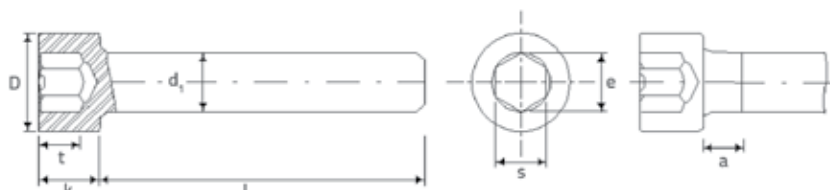
Slika 2. Detalji vijaka
