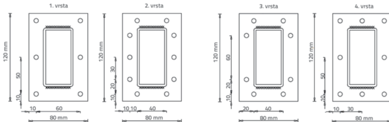
Slika 1. Vrste priključaka
