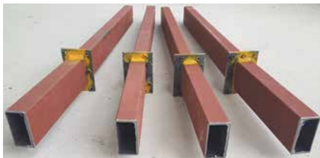
Slika 4. Detalji ispitnih uzoraka
