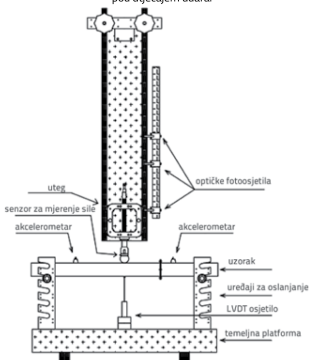
Slika 5. Shema sustava za ispitivanje
