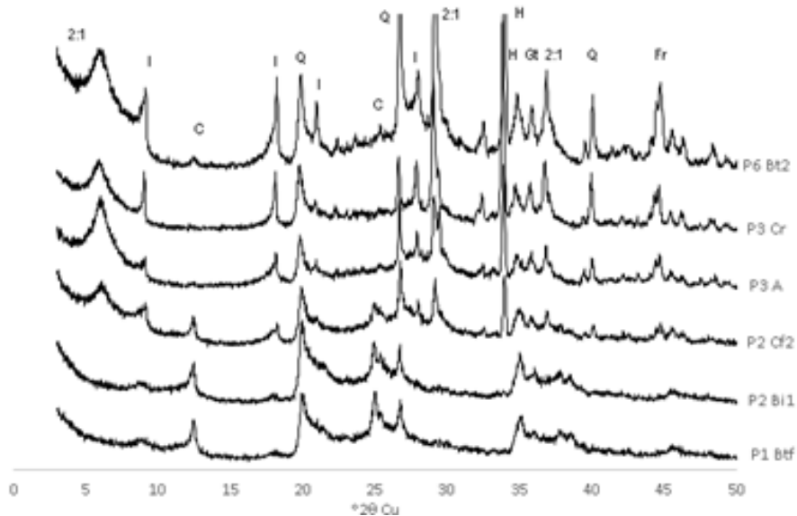
Figura 6: Mineralogia da fração argila de amostras dos solos de Gilbués, PI. 2:1- mineral da argila 2:1; I- Illita; Q- Quartzo; H- Hematita; C- caulinita; Gt- Goethita; Fr- Ferrihidrita.
