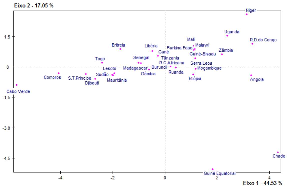
Figura 12 Representação dos indivíduos no plano principal [1,2] para o ano 2004
