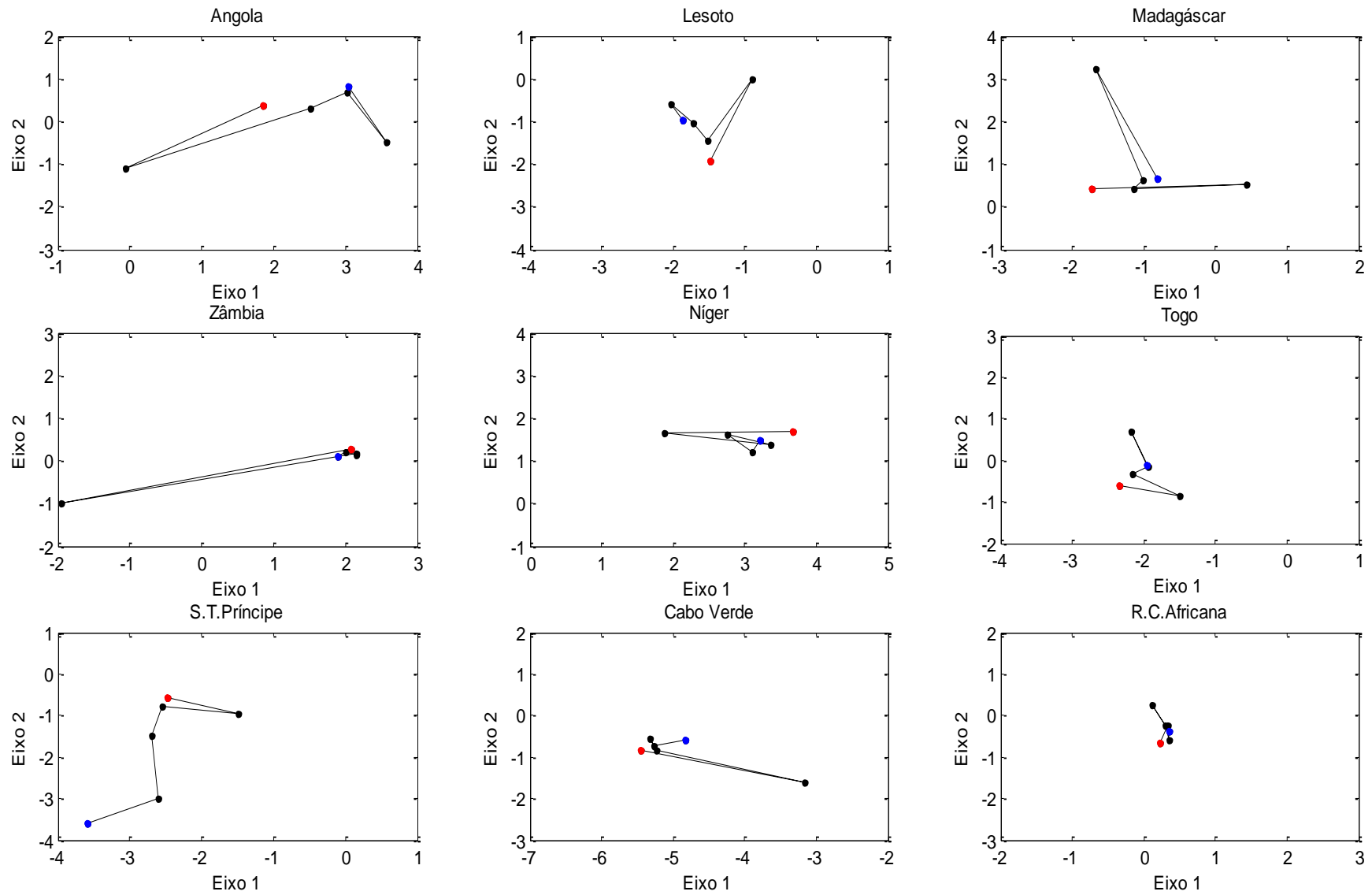
Figura 23 Trajetórias de cada um dos países (1º critério). Continuação
