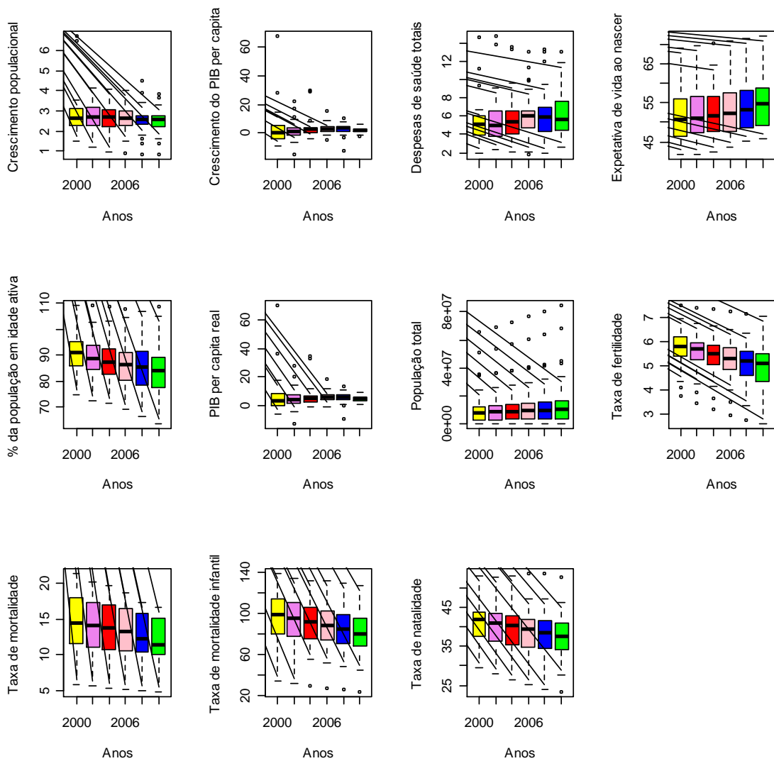
Figura 3 Boxplots das variáveis
