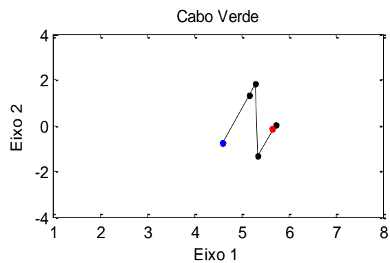
Figura 27 Trajetórias de cada um dos países (2º critério). Continuação
