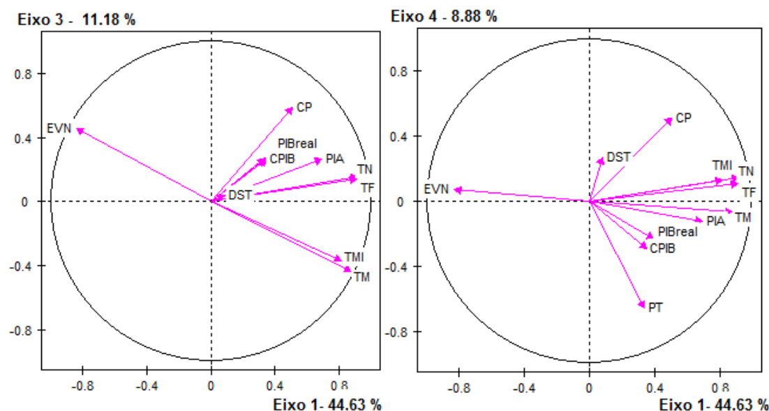
Figura A. 4 Círculo de correlações no plano principal [1,3] e no plano principal [1,4] do ano 2002
