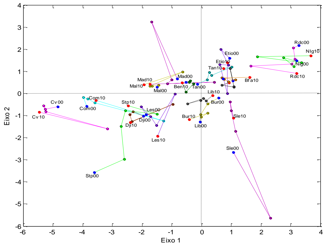
Figura 31 As trajetórias que revelam maior grau de oposição relativamente ao 2º eixo
