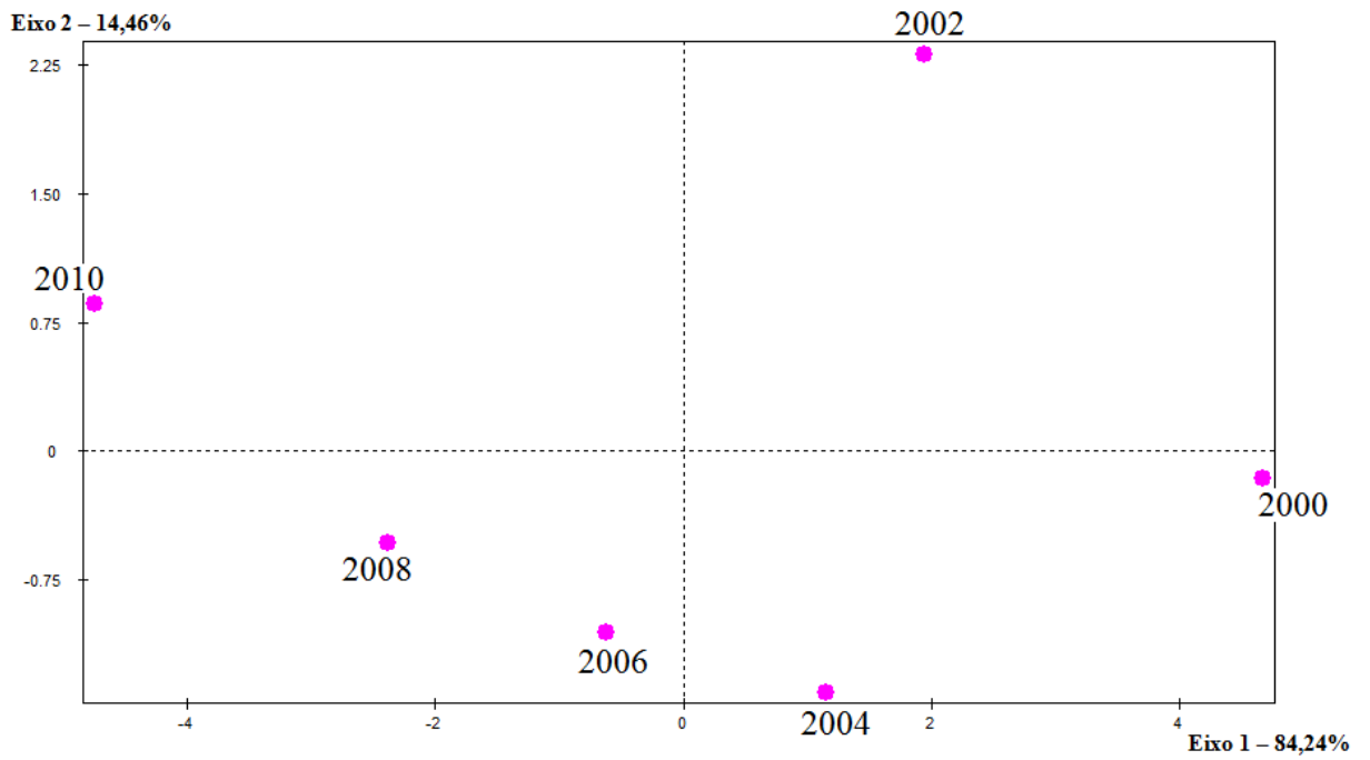
Figura 5 Imagem euclidiana da inter-estrutura.
