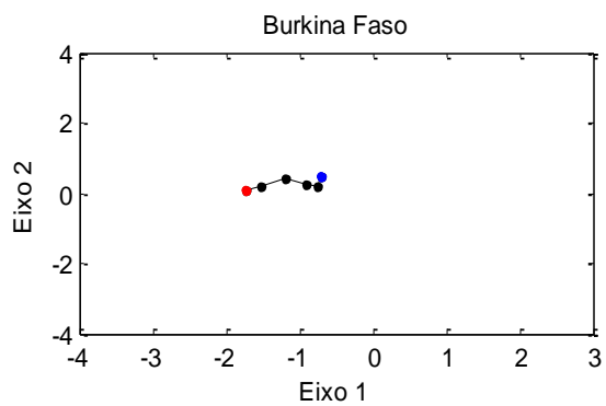
Figura 28 Trajetórias de cada um dos países (2º critério). Continuação
