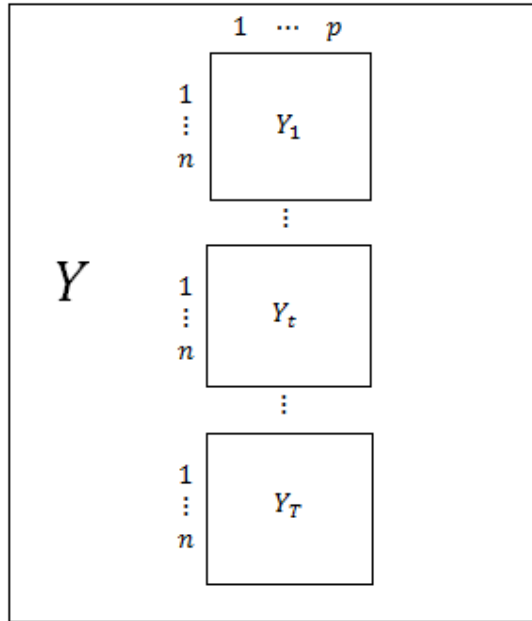
Figura 2 Sobreposição dos quadros de dados centrados.
