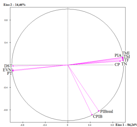
Figura 4 Círculo de correlações das variáveis no plano 1-2 (inter-estrutura da DACP)
