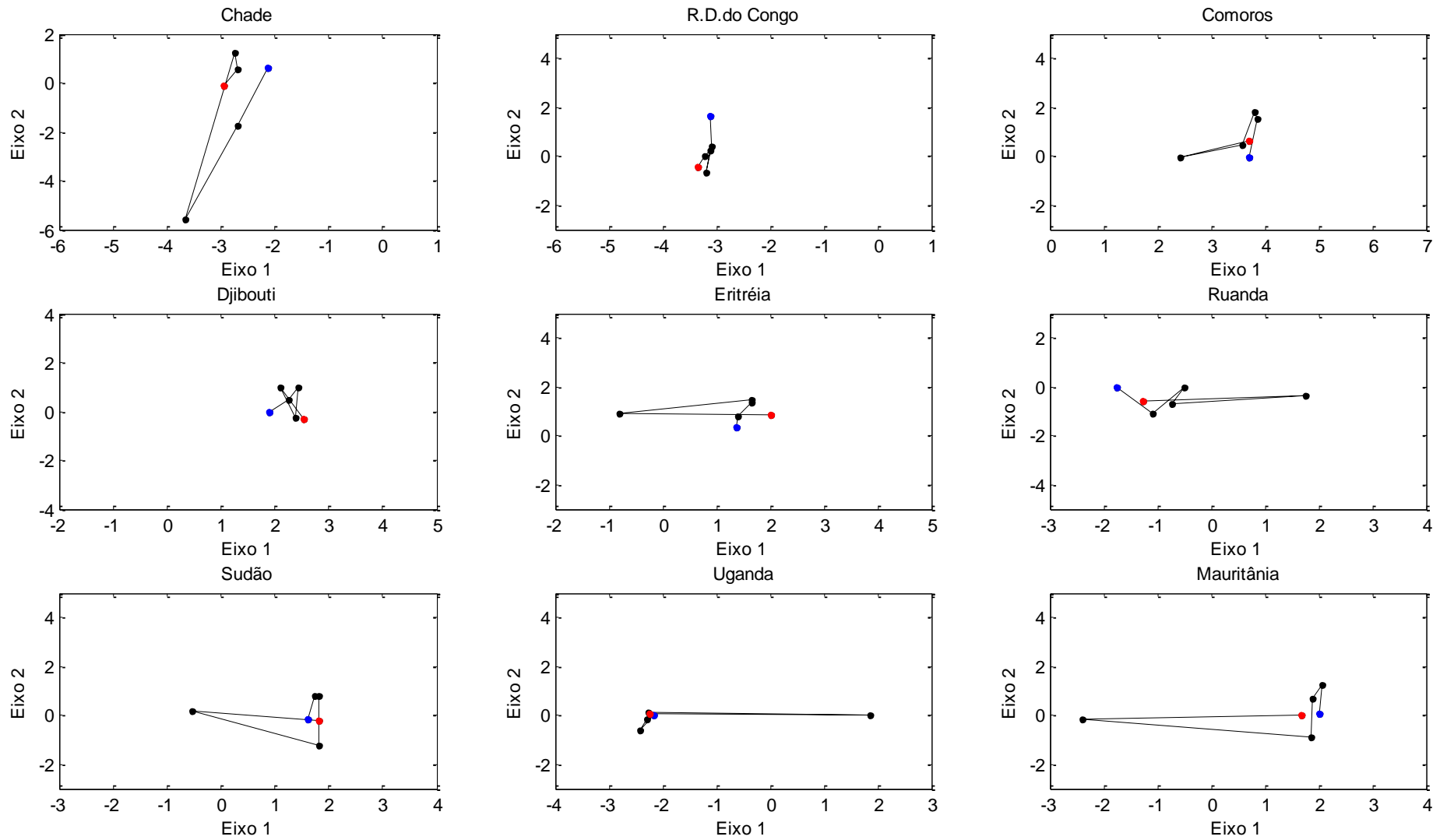
Figura 26 Trajet rias de cada um dos pa ses (2  crit rio)
