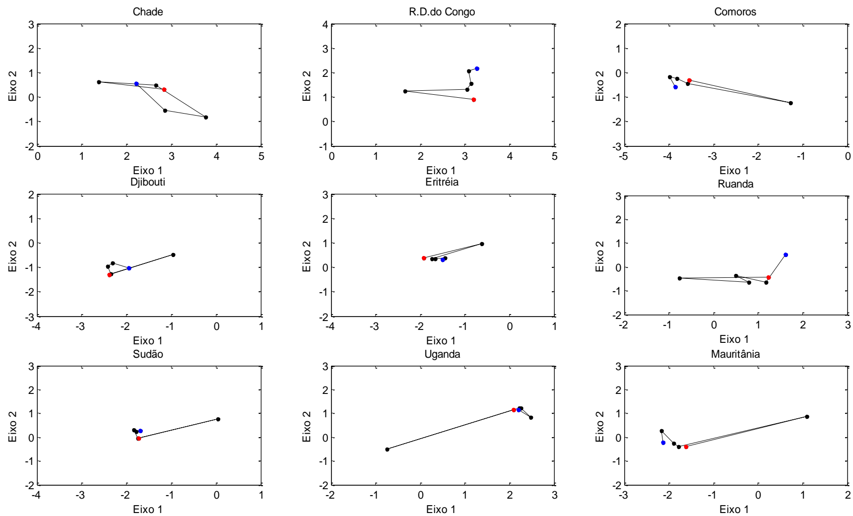
Figura 22 Trajet\u00f3rias de cada um dos pa\u00edses (1\u00b0 crit\u00e9rio)
