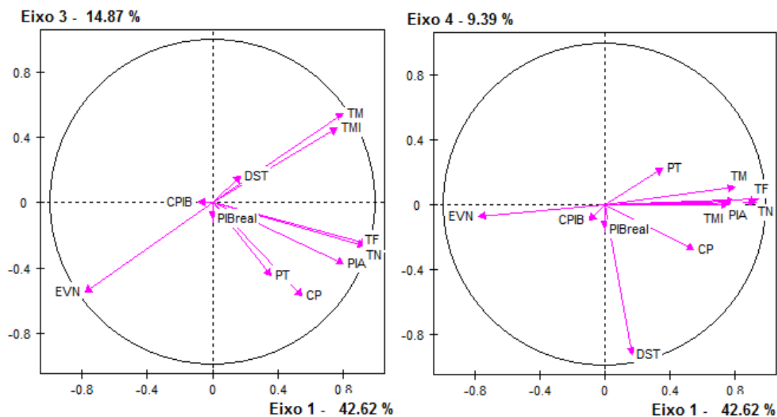
Figura A. 10 Círculo de correlações no plano principal [1,3] e no plano principal [1,4] do ano 2006
