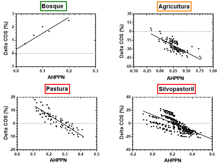
Figura 4.9: Cambios en los contenidos de C en el suelo (delta COS) de cada uno de los manejos y usos simulados en función de la apropiación humana de la productividad primaria neta (AHPPN). El delta COS (%) se calculó como la diferencia porcentual entre el valor simulado al final de la corrida y el valor simulado para la situación de bosque pristino. La AHPPN se calculó como la diferencia relativa entre la PPN original y la PPN remanente, es decir, la que surge de la diferencia entre la PPN del sistema actual y la cosechada (ecuaciones 2 y 3). Los primeros 4 paneles representan los usos y manejos del sitio más seco, mientras que en el sitio más humedo se encuentran representados por los últimos 4 paneles.
