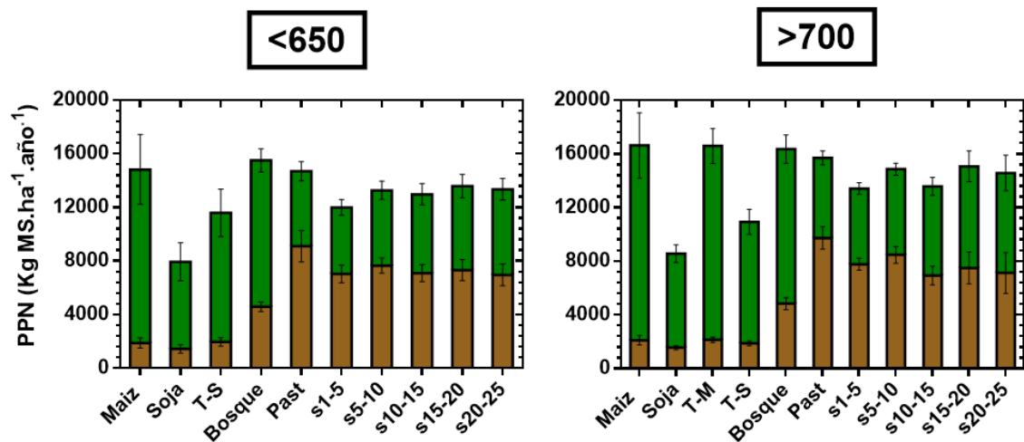
Figura 3.5: Productividad primaria neta (PPN) promedio anual de las distintas coberturas y usos del suelo del Departamento de Anta, Salta, para dos sitios con diferente precipitación media anual. La productividad primaria neta subterránea (PPNS) promedio anual se indica en color marrón, mientras que la productividad primaria neta aérea (PPNA) promedio anual se encuentra indicada en color verde. Las líneas sobre las barras indican el desvío estándar interanual (2001-2010). Coberturas y usos del suelo: Maiz, Soja, Trigo-Soja (T-S), Bosque, Pasturas (Past), y Sistemas silvopastoriles con distinta cobertura arbórea (S1-5, S5-10, S10-15, S15-20 y S20-25).
