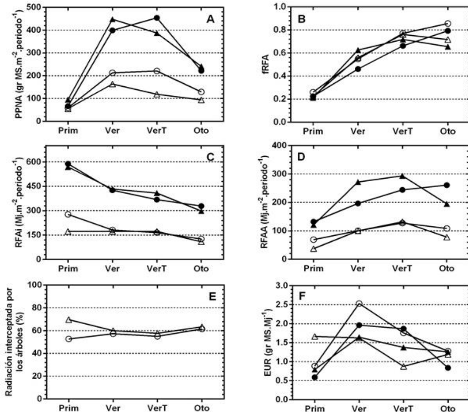
Figura 2.4: (A) Productividad primaria neta aérea (PPNA), (B) Fracción de radiación fotosintéticamente activa interceptada por la vegetación (fRFA), (C) Radiación fotosintéticamente activa incidente (RFAi), (D) Radiación fotosintéticamente activa absorbida (RFAA), (E) radiación interceptada por el árbol, y (F) Eficiencia de uso de la radiación (EUR) de pasturas de Gatton panic ( Megathyrus maximus ). Las variables fueron medidas en primavera (Prim), verano (Ver), verano tardío (VerT) y otoño (Oto) en dos sitios: húmedo (H) y seco (S). Todas las variables medidas mostraron un claro patrón estacional, aunque la radiación interceptada por los árboles mostró la menor variabilidad a lo largo del periodo de crecimiento. Los puntos negros y los triángulos corresponden al tratamiento sin árbol (NA) y los puntos blancos y los triángulos corresponden al tratamiento con árboles de Guayacán ( Caesalpinia paraguariensis ) (A). Los puntos corresponden al sitio húmedo (H) y triángulos al sitio seco (S).
