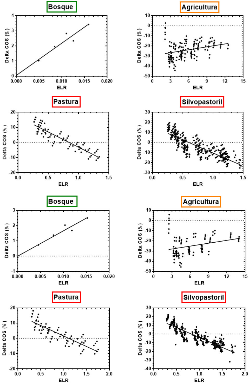
Figura 4.11: Cambios en los contenidos de C en el suelo (delta COS) de cada uno de los manejos y usos simulados en función de un indicador de la presión ambiental (ELR). El delta COS (%) se calculó como la diferencia porcentual entre el valor simulado al final de la corrida y el valor simulado para la situación de bosque prístino. El ELR se calculó como el cociente entre la energía no renovable (natural o antrópica) y la energía renovable implicada en la producción de commodities. Los primeros 4 paneles representan los usos y manejos del sitio más seco, mientras que en el sitio más húmedo se encuentran representados por los últimos 4 paneles.
