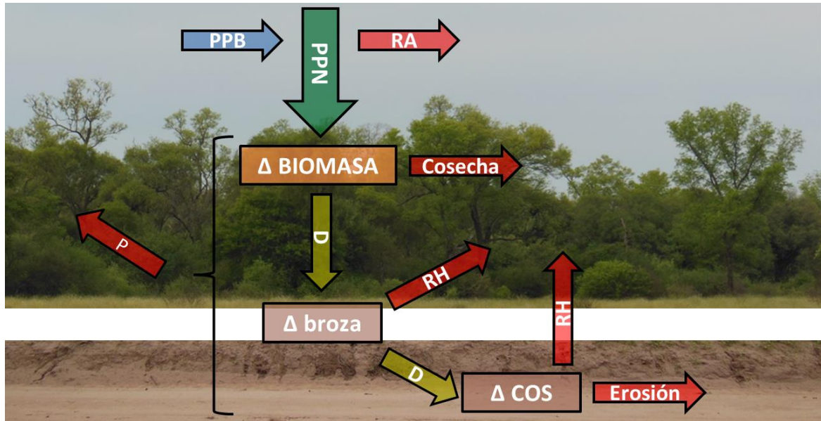
Figura 1.4: Reservorios y flujos de entrada y salida del C en un esquema simplificado de la dinámica del carbono en un ecosistema forestal del chaco seco argentino. El carbono se acumula en el suelo ( \Delta broza y \Delta COS) a través del carbono de origen vegetal (biomasa aérea y subterránea muerta) no consumido por los microorganismos, que llega al suelo en forma de detritos (D). El resto del carbono puede perderse hacia la atmósfera por fuego (P), ser respirado por los microorganismos del suelo (RH) (descomposición), o mediante la erosión del suelo. El compartimiento \Delta Biomasa incluye tanto la aérea como la subterránea, la cual puede ser cosechada o consumida por los herbívoros. Adaptado de Gower, (2003).
