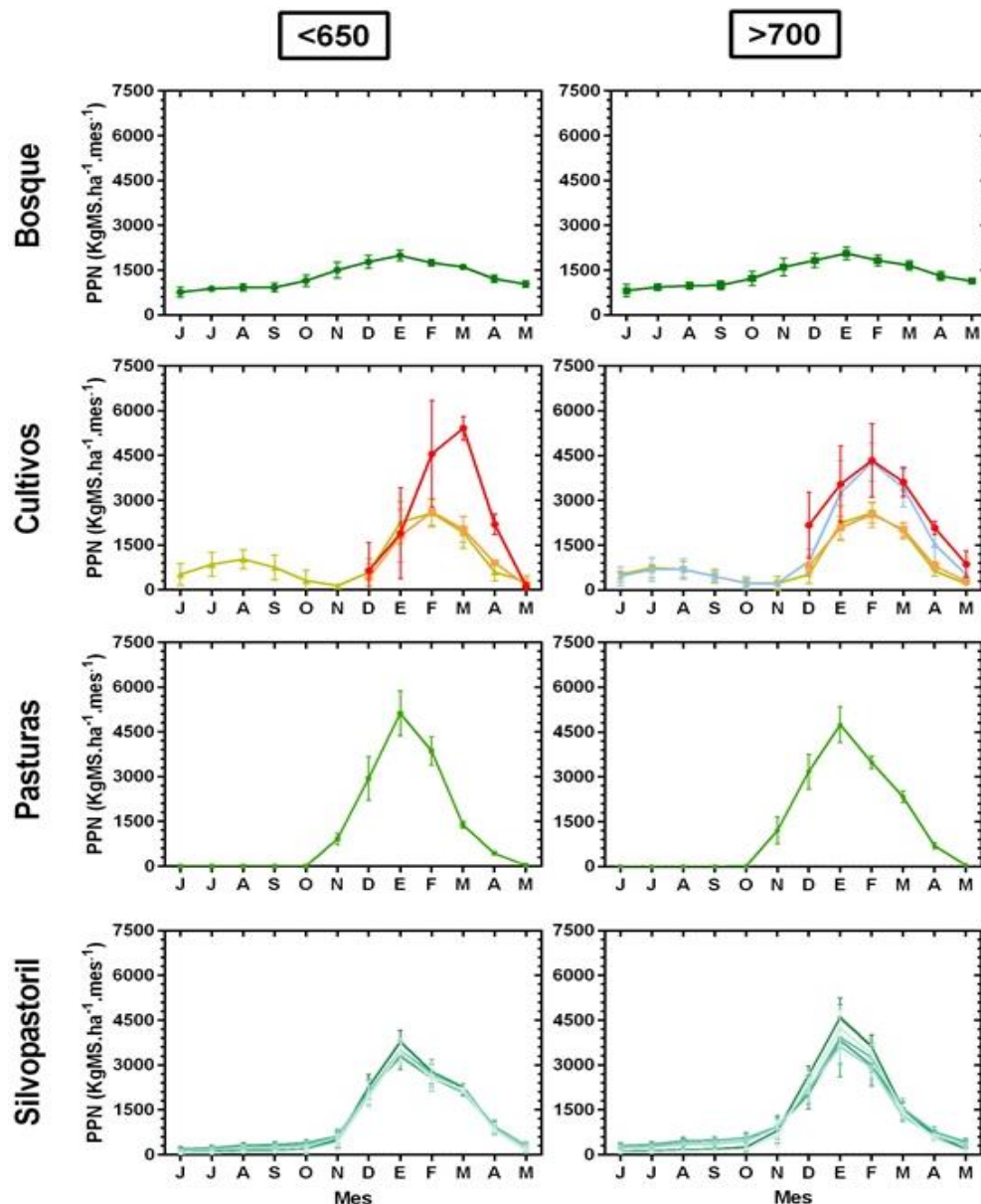
Figura 3.8: Productividad primaria neta (PPN) promedio mensual de las distintas coberturas y usos del suelo del Departamento de Anta, Salta, para dos sitios con diferente precipitación media anual. Las líneas sobre las barras indican el desvío estándar interanual (2001-2010).
