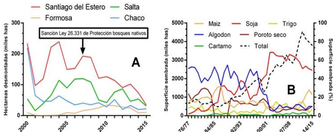
Figura 1.3: (A) Superficie desmontada (en miles de hectáreas) entre los años 2000 y 2015 en la ecoregión argentina del Chaco Seco para las cuatro provincias más representativas (Santiago del Estero, Salta, Chaco y Formosa), en base a los desmontes registrados por el proyecto “Monitoreo de desmontes en el Chaco Seco” ( http://monitoreodesmonte.com.ar/ ). A partir de 2007 (año en el cual fue sancionada la Ley N° 26.331 de Protección de los Bosques Nativos) se observa una tendencia decreciente en las áreas desmontadas. (B) Superficie sembrada total y de los principales cultivos de la región (maíz, soja, trigo, algodón, poroto seco y cártamo) entre los años 1976 y 2015 (en miles de hectáreas), en base a los registros obtenidos del Sistema Integrado de Información Agropecuaria (SIIA) del Ministerio de Agroindustria de la Nación.
