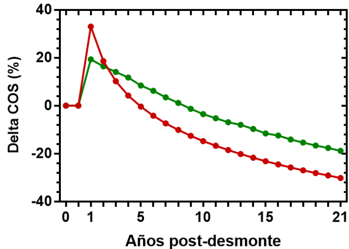
Figura 4.12: Cambios en los contenidos de C en el suelo (delta COS) en sitios agrícolas respecto del bosque prístino en función del tiempo transcurrido luego del desmante. En línea roja se muestra el modelo ajustado por Villarino et al. (2017) en base a 21 muestras de suelo para una profundidad de 0-30 cm. En verde se muestra el comportamiento promedio del delta COS (%) para las principales rotaciones agrícolas de la región (Mosciaro, comunicación personal), simuladas con el modelo CENTURY.
