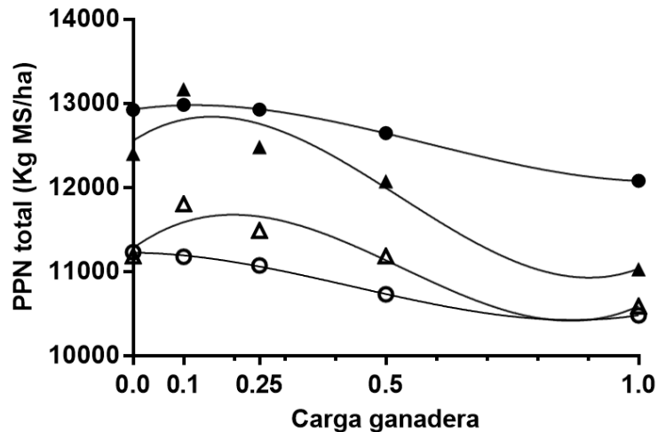
Figura 4.8: Variación promedio en la PPN total (en Kg MS/ha.ano) en respuesta al incremento en la carga ganadera en pasturas puras (círculos) y sistemas silvopastoriles (triángulos). Los símbolos negros indican el sitio más húmedo y los vacíos el sitio más seco.
